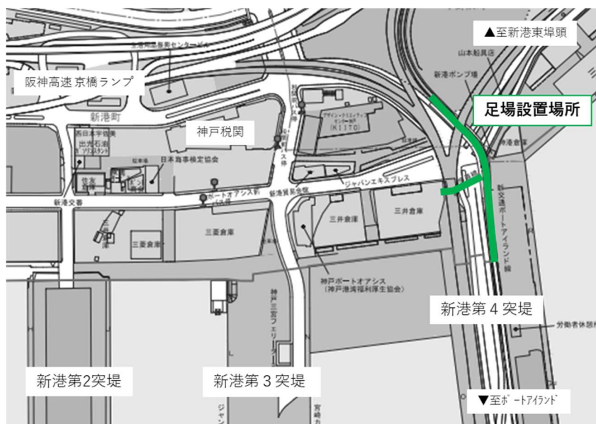
位置図(1/2)
