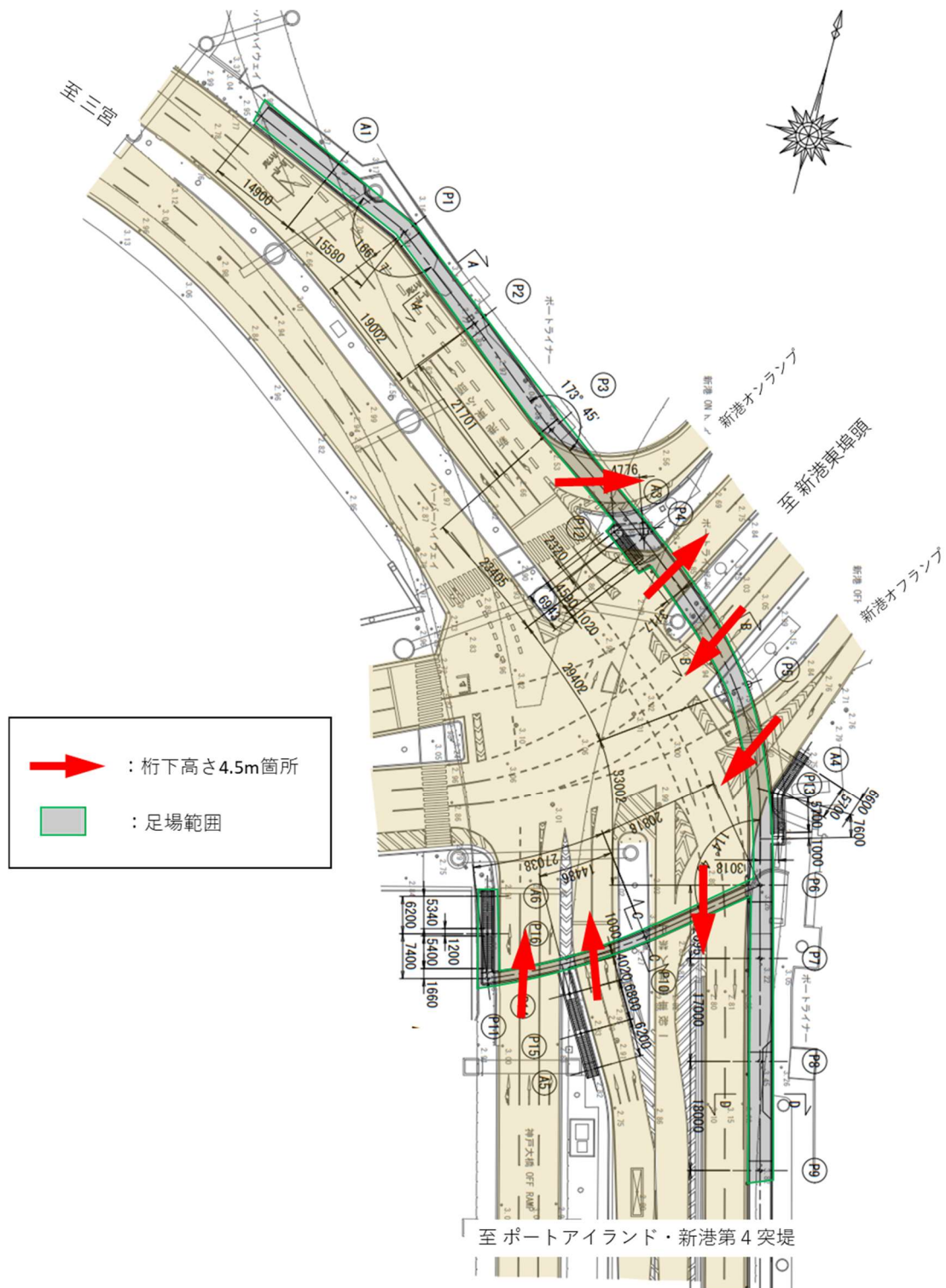
位置図(2/2)
