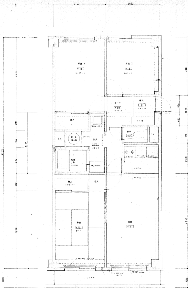
⑧ 型平面図 1:50
