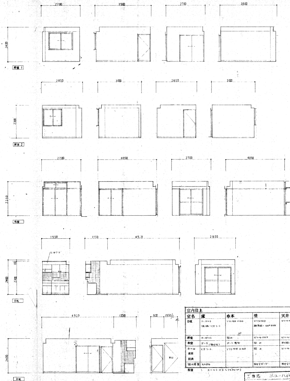
展開図 1:
