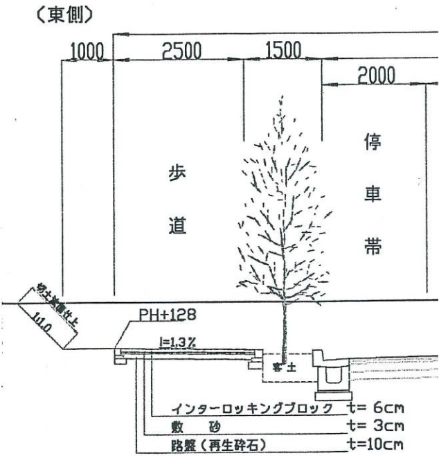
断面図 1/100
