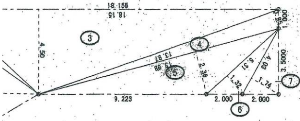
道路求積図 S=1:200
