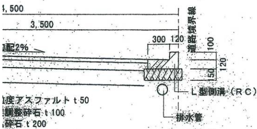
断面図 S=1:50
