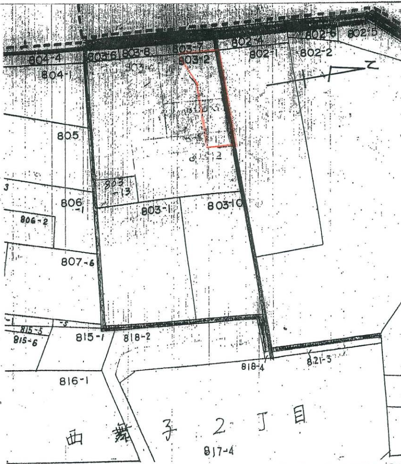
界限図
