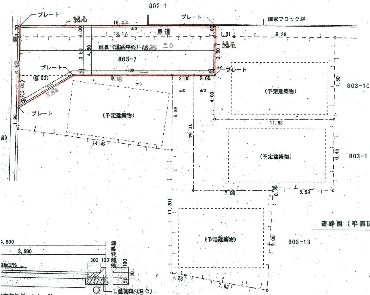
界限図
