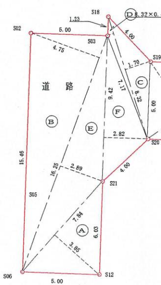
道路三斜求積図
