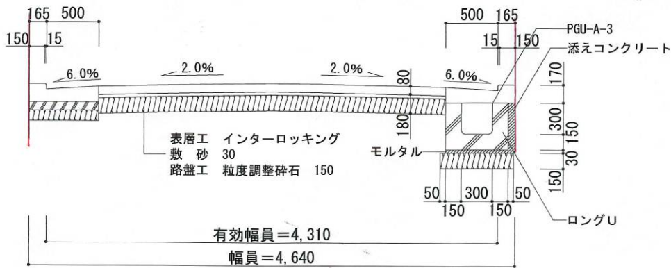
A~A' 断面図 S. 1 : 50
