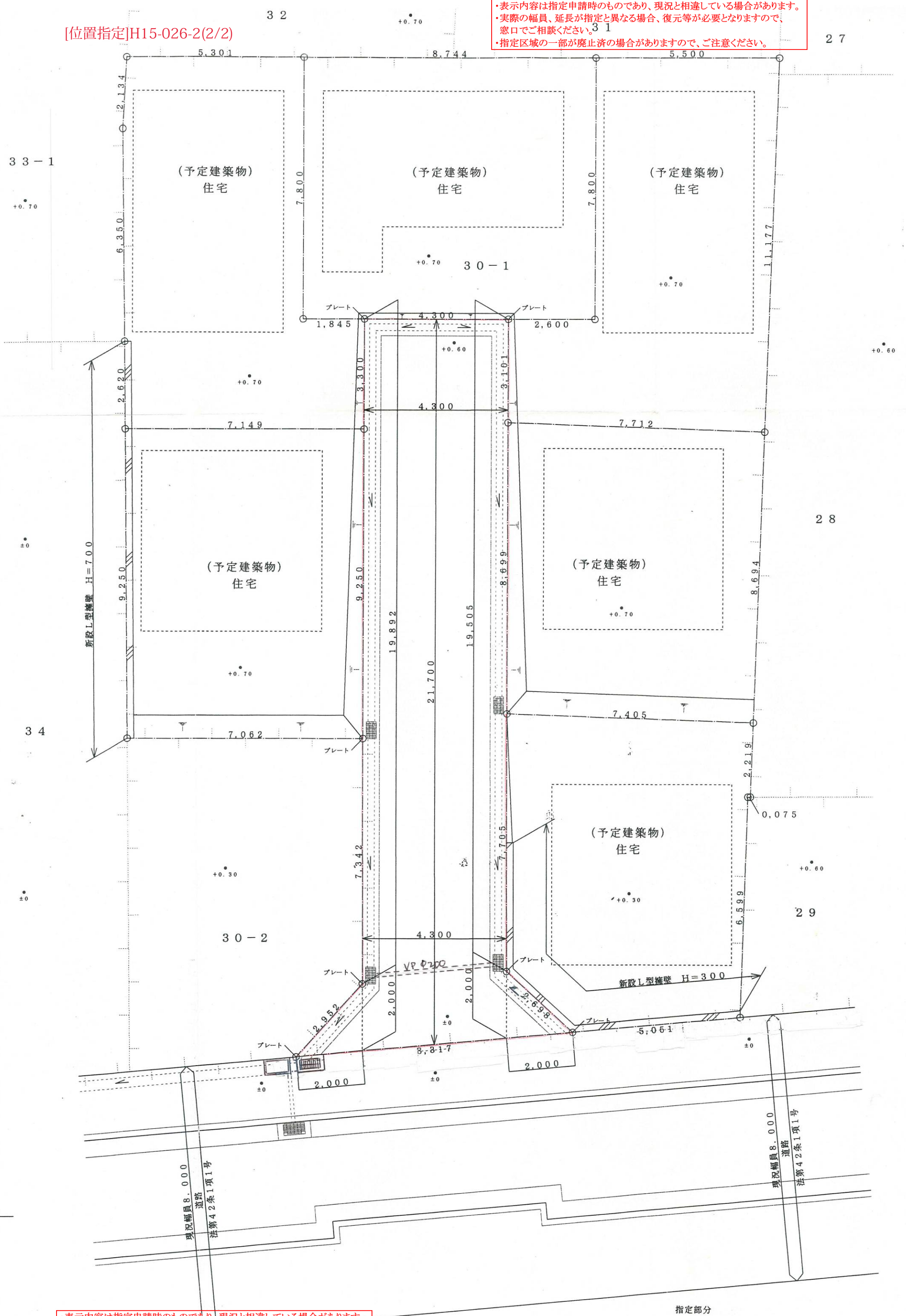
道路指定図 1/100
