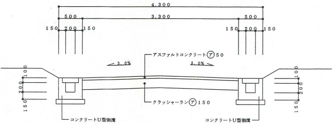
標準横断面図 1/50
