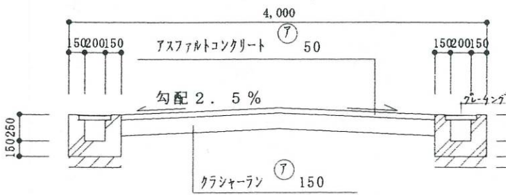
断面図 1:50
