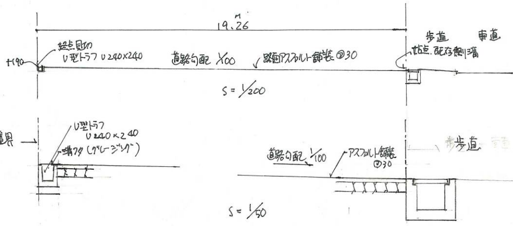
B-B 断面図
