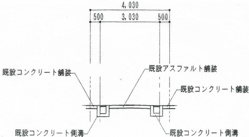
1-1道路断面図 S=1:100
