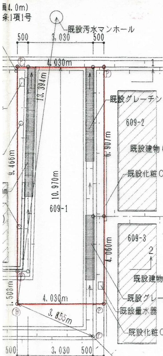
道路平面図 S=1:100
