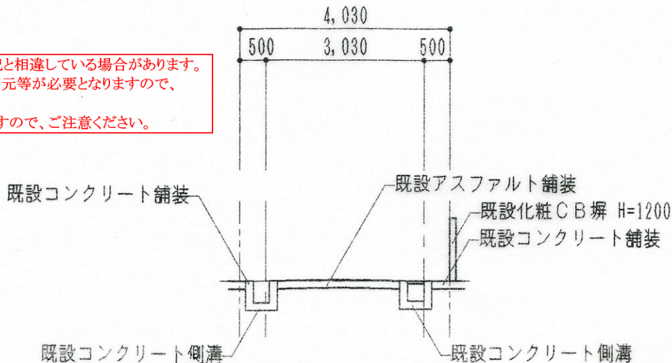
2-2道路断面図 S=1:100
