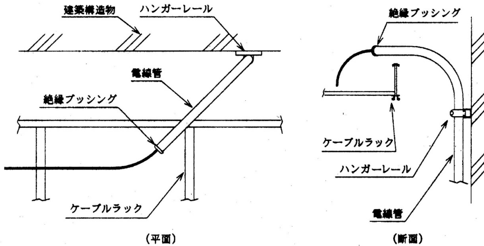
図 4-3-9 金属管引出し参考図 (アルミ製ケーブルラック)
