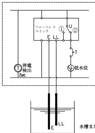
図4-2-5フロートレス液面スイッチ回路参考図
