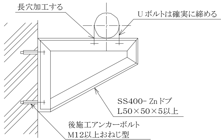
図 3-4-5 垂直荷重支持①
