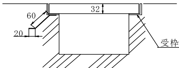
図 3-2-4 グレーチング蓋図(施工例)
