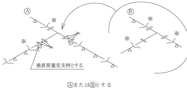
図 3-4-4 分岐
