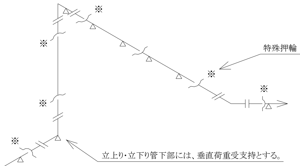
図 3-4-2 曲管
