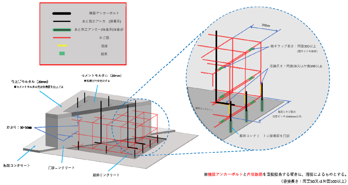
図 3-3-2 静荷重形基礎要領図
