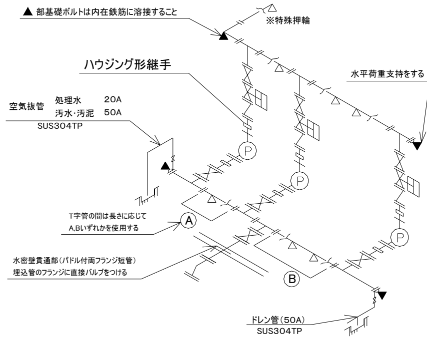
図 3-4-3 ヘッダー管
