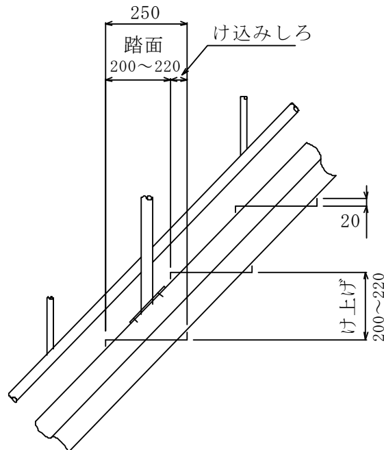
図 3-2-1 階段標準図
