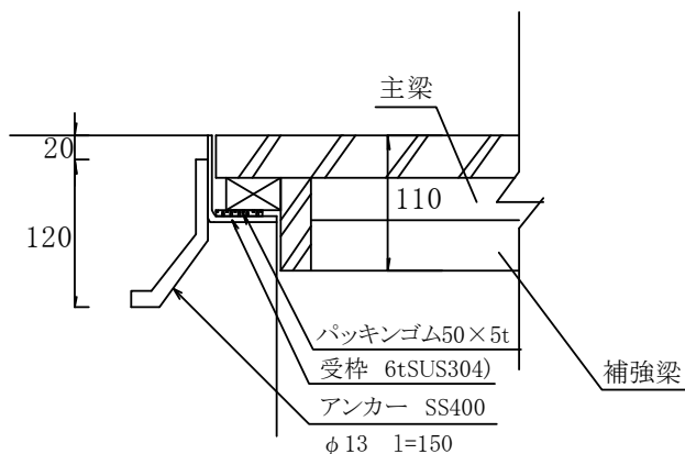
図 3-2-6 合成木材蓋 (参考図)
