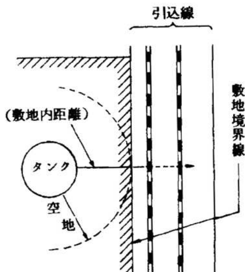
例図3(告示第4条の2の2第3号)
