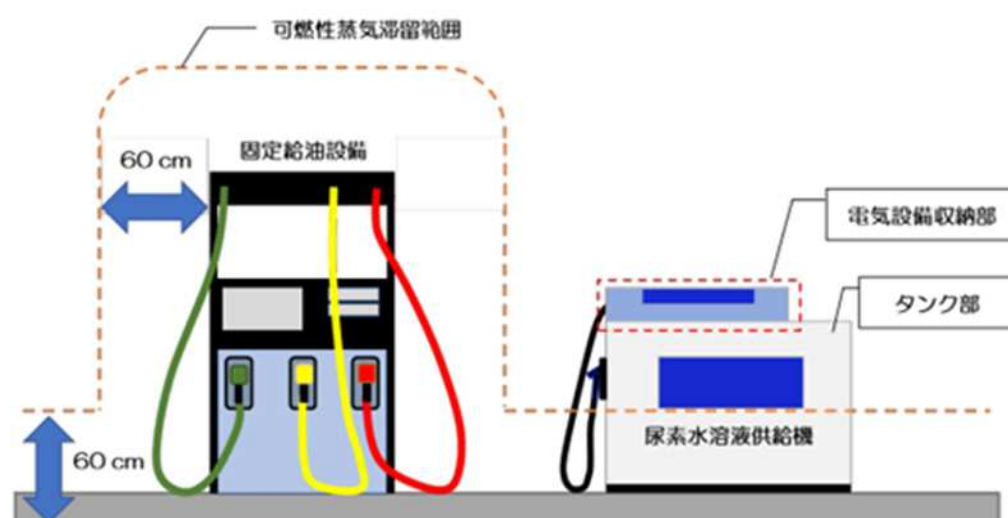
尿素水溶液供給機（電動ポンプにより払い出すタイプ）
