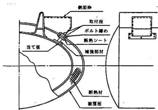
図 2-7-10 外板の下部に補強部材を設け、側面枠と補強部材をボルト締めにより接合する場合の取付方法
