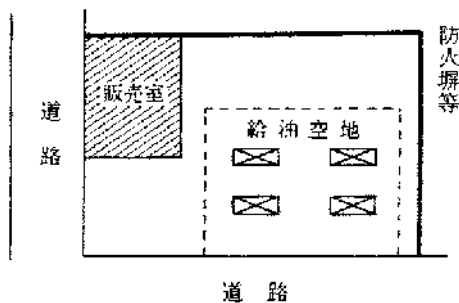
〔二方開放とならない例〕
