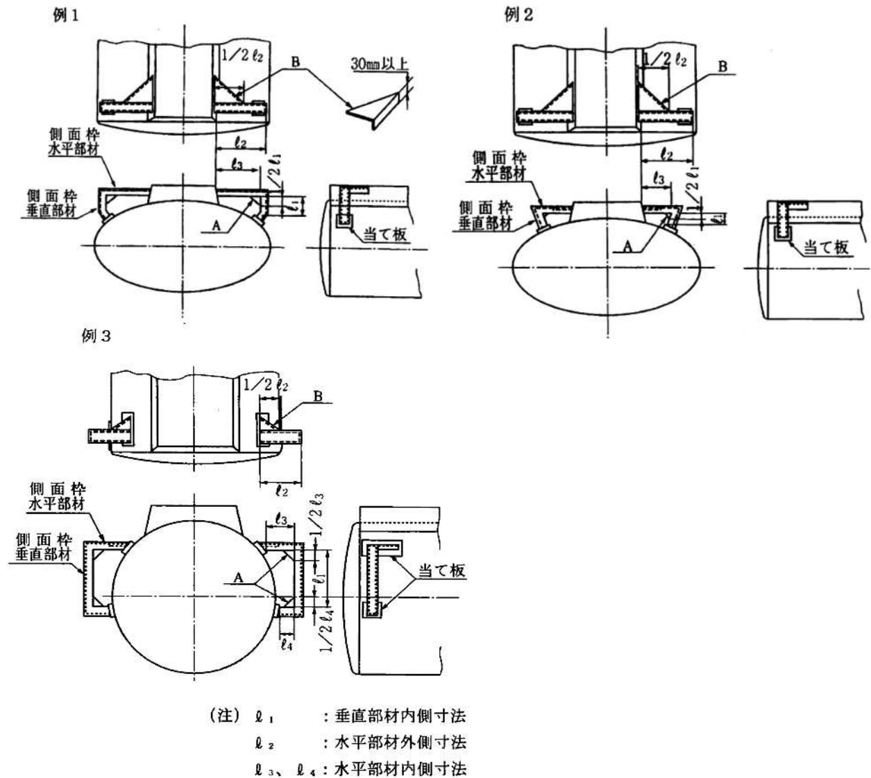
図 2-7-1 枠形の側面枠の構造
