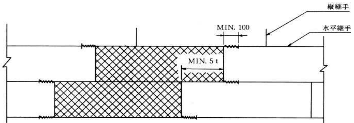
側板複数の取替
