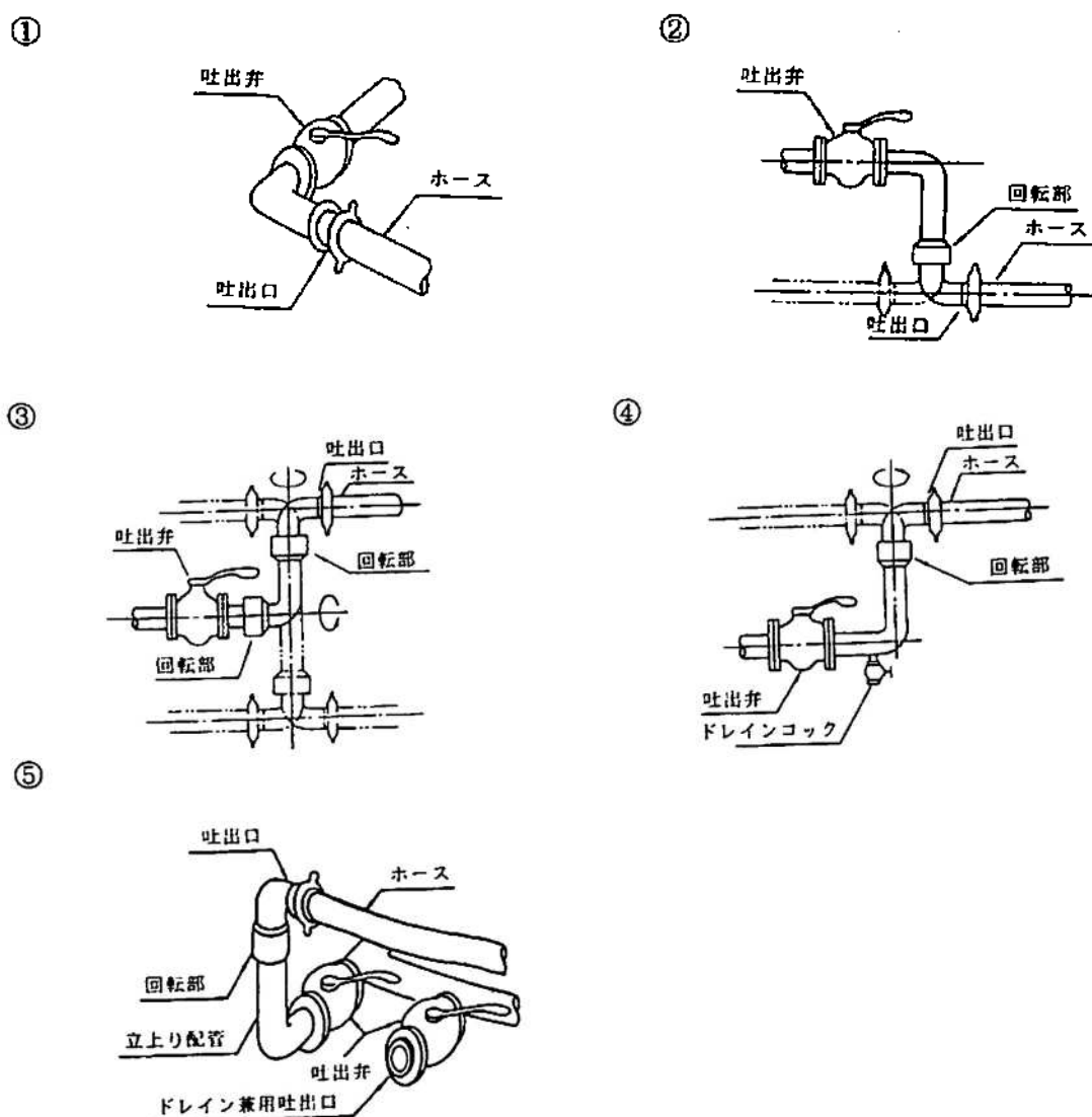
図 2-14-2 配管先端部の構造
