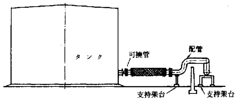
立面図
