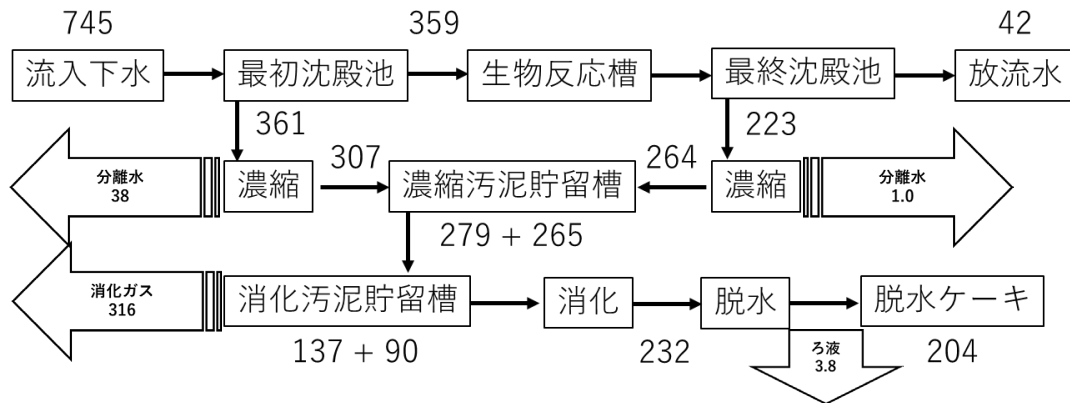
図2 CODクロム換算による処理工程でのエネルギー収支 (GJ/日)
