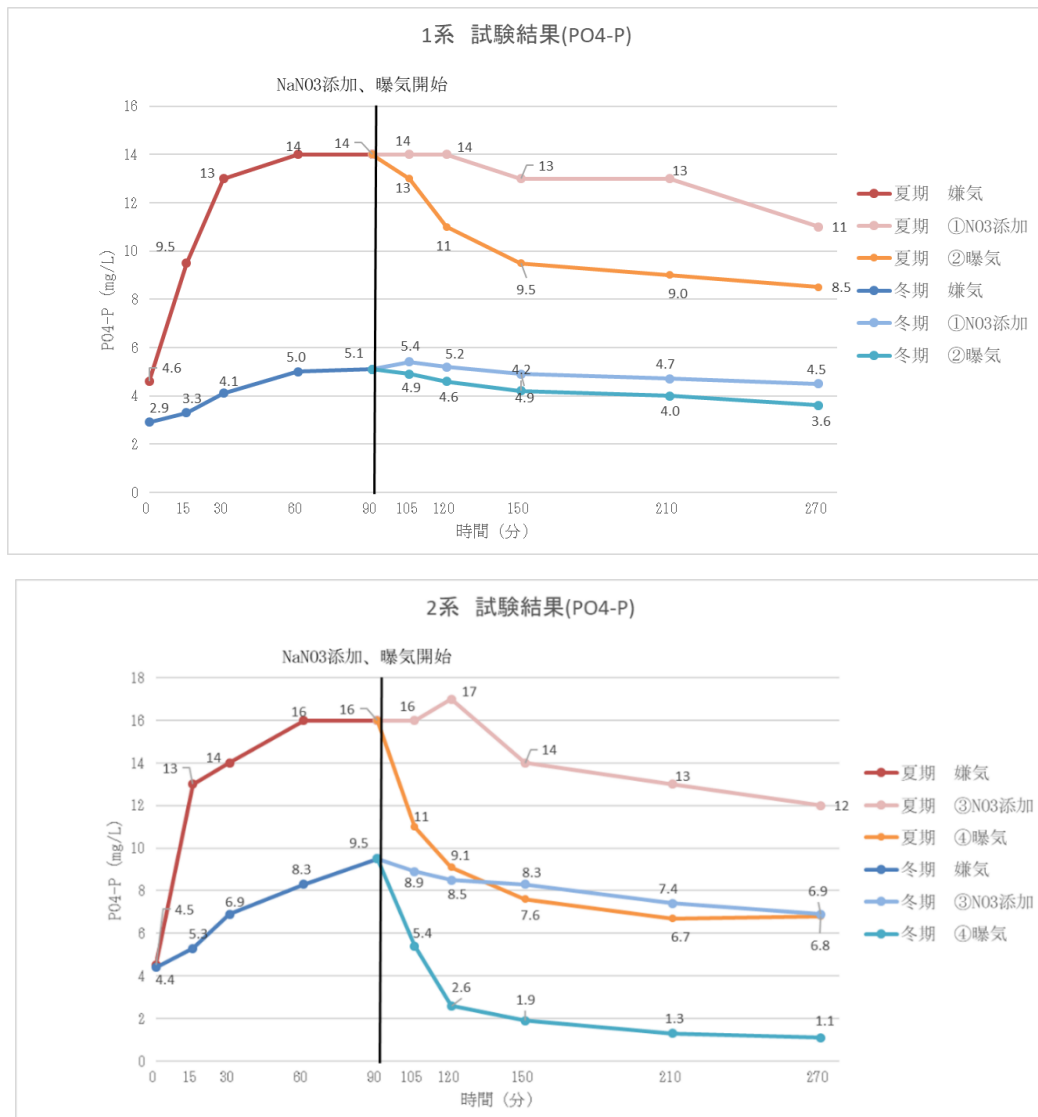
図-2 本場 1 系、2 系でのりん酸態りんの挙動
