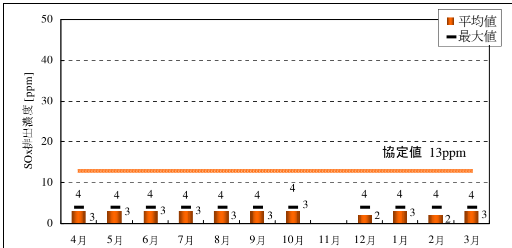
図 6-9 神戸発電所 3 号機の SOx 排出濃度
