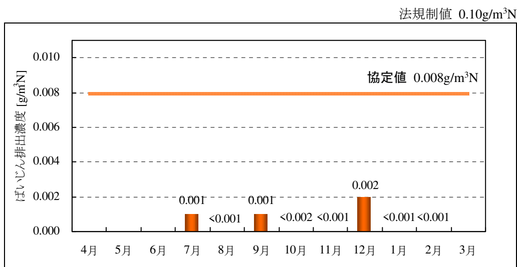
図 6-18 神戸発電所 1 号機のばいじん排出濃度
