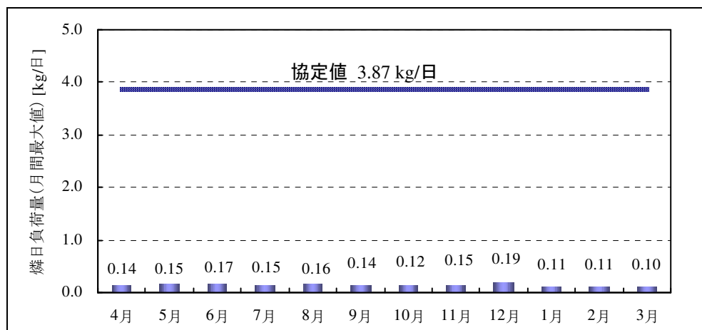
図 8-4 T-P の日負荷量 (月間最大値)
