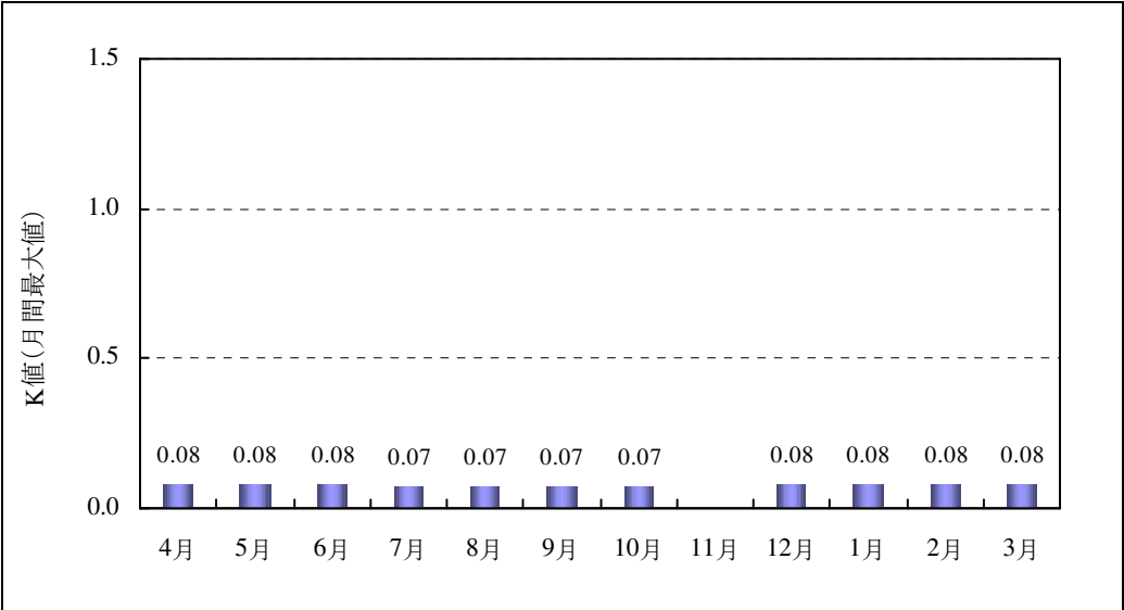
図 2-3 神戸発電所 3 号機の K 値（月間最大値）
