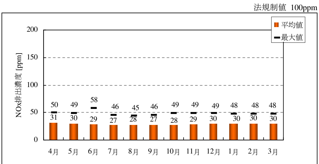
図 6-13 棒鋼工場加熱炉の NOx 排出濃度
