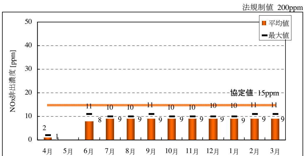
図 6-17 神戸発電所 4 号機の NOx 排出濃度
