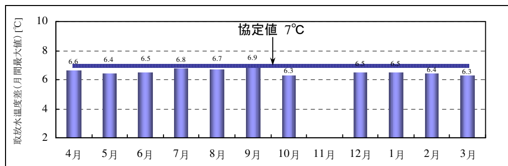
図 8-7 神戸発電所 2 号機の取放水温度差（月間最大値）
