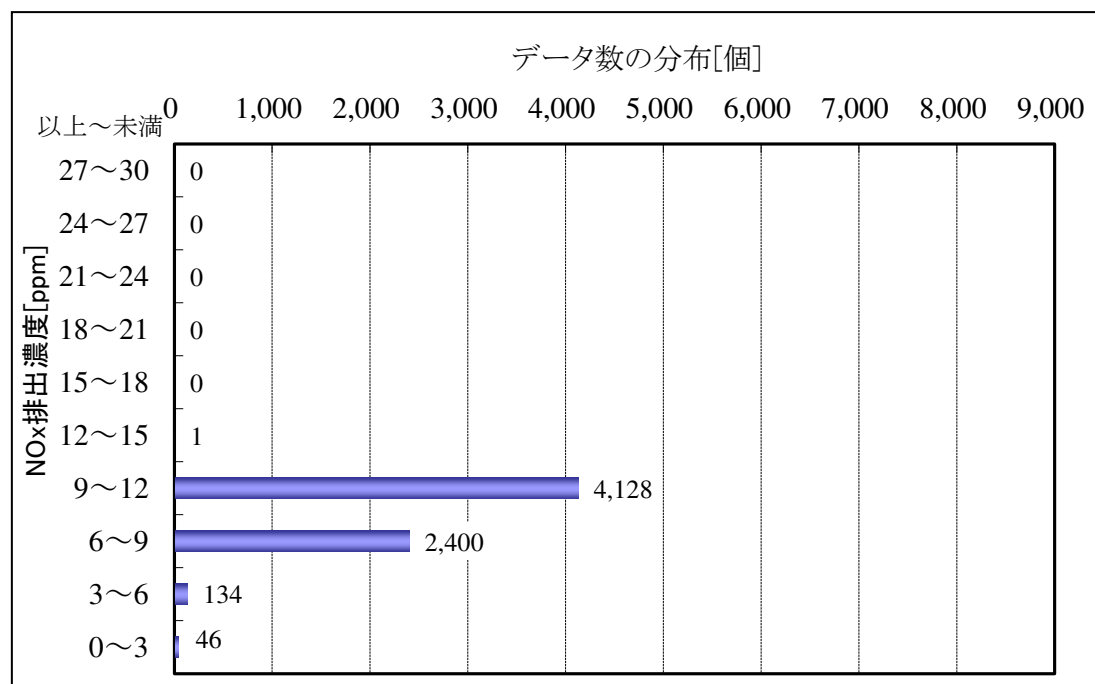
図 1-10 神戸発電所 3 号機の NOx 排出濃度の分布 (1 時間値)
