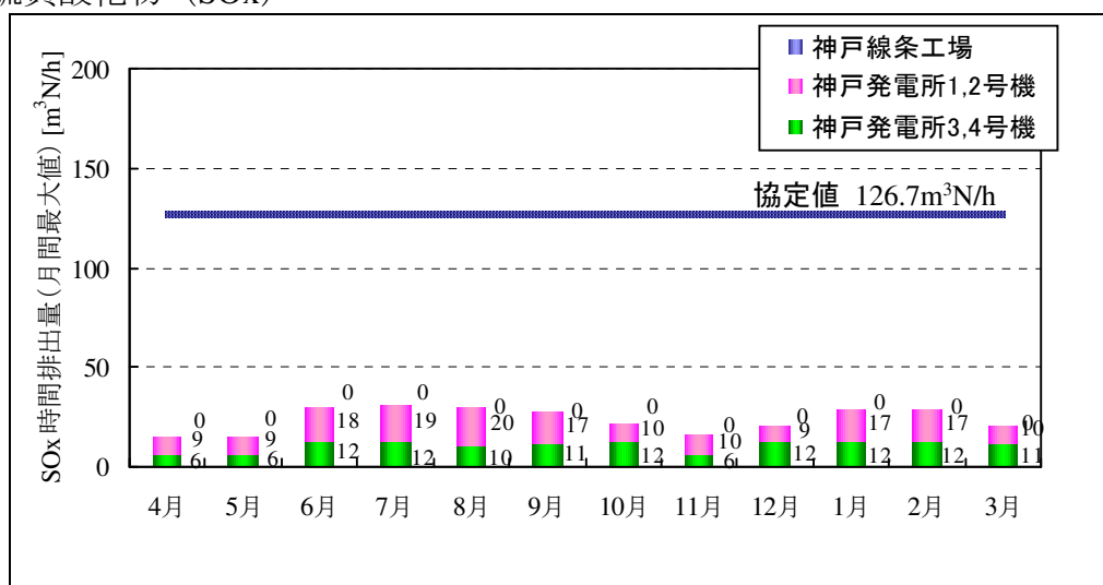
図 3-1 事業場からの SO x 時間排出量（月間最大値）
