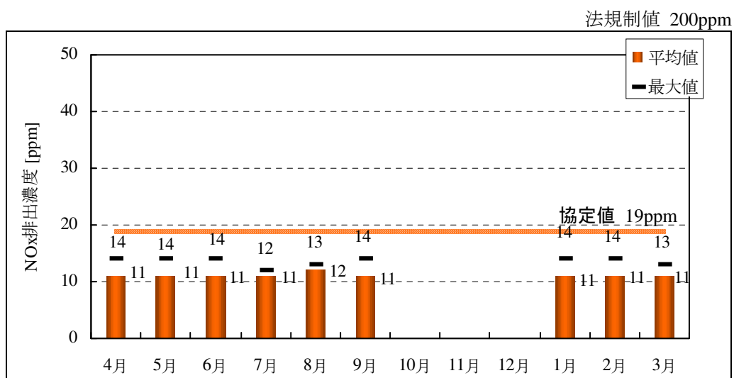
図 6-15 神戸発電所 2 号機の NOx 排出濃度
