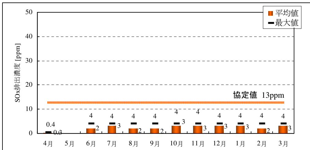
図 6-10 神戸発電所 4 号機の SOx 排出濃度
