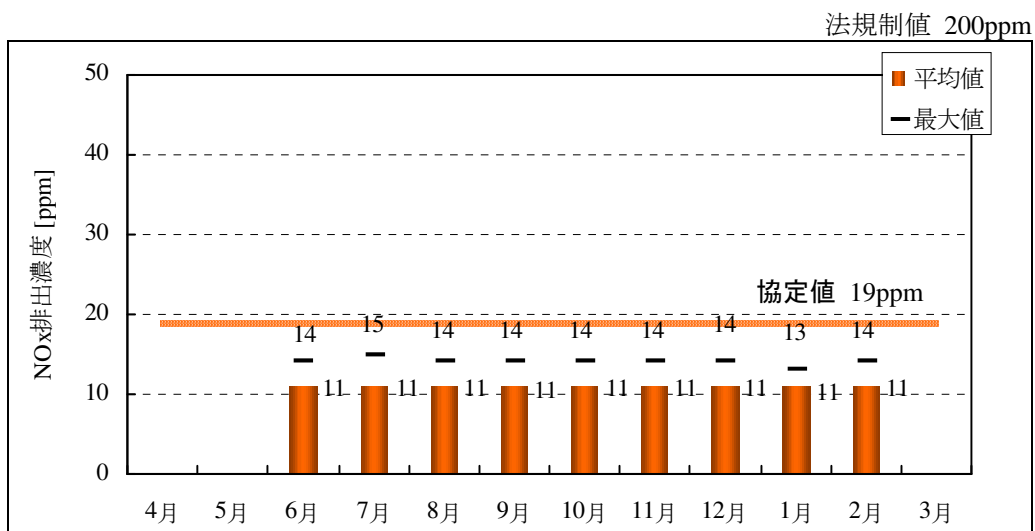
図 6-14 神戸発電所 1 号機の NOx 排出濃度
