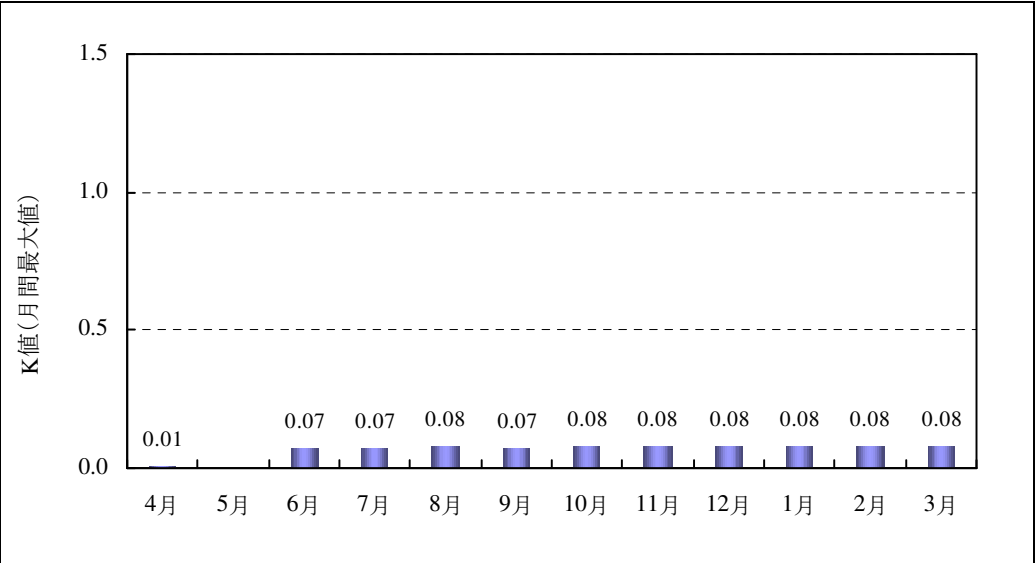
図 2-4 神戸発電所 4 号機の K 値（月間最大値）
