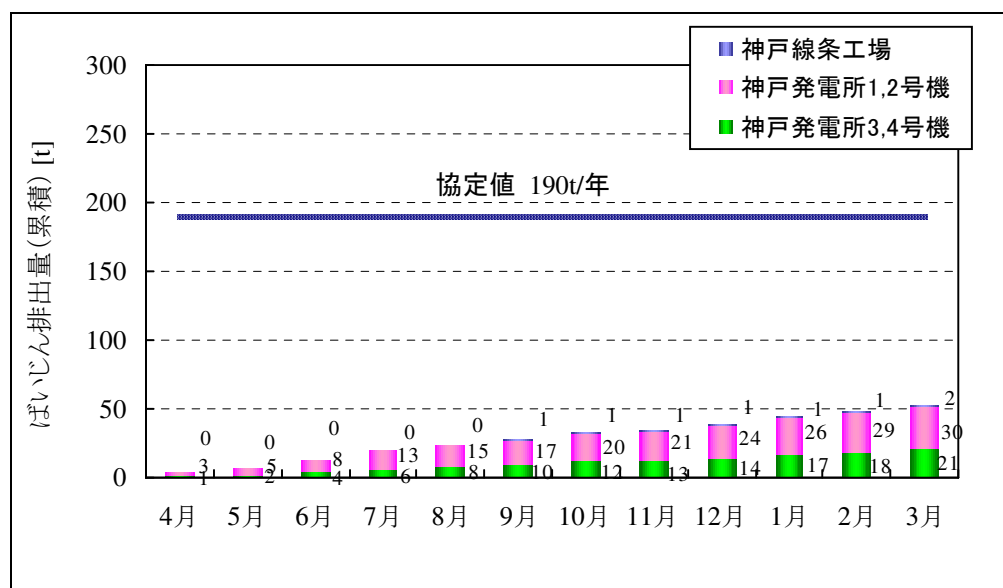
図 3-6 事業場からのばいじん排出量（累積）
