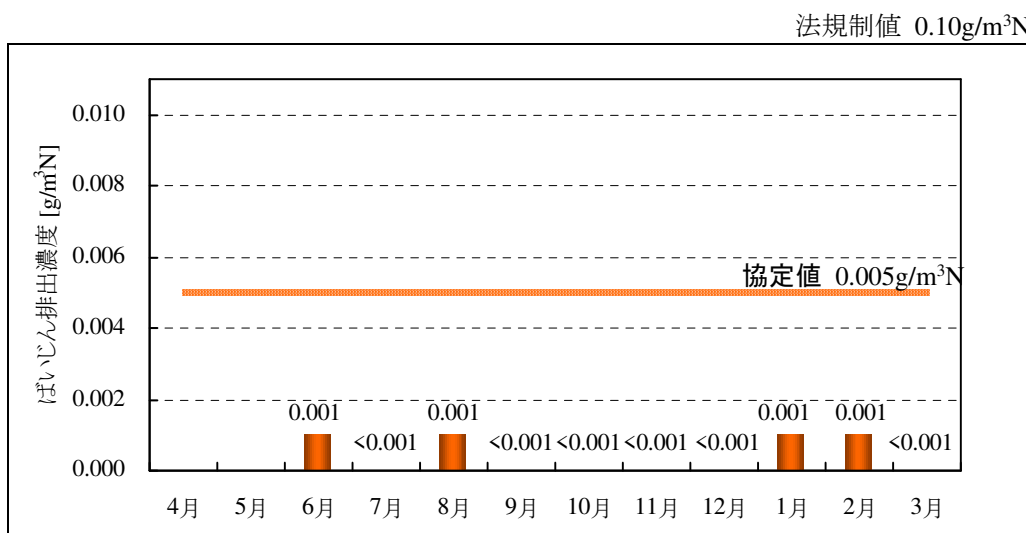
図 6-21 神戸発電所 4 号機のばいじん排出濃度
