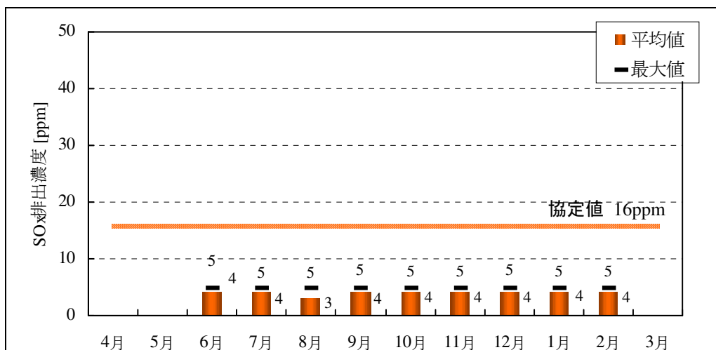
図 6-7 神戸発電所 1 号機の SO x 排出濃度
