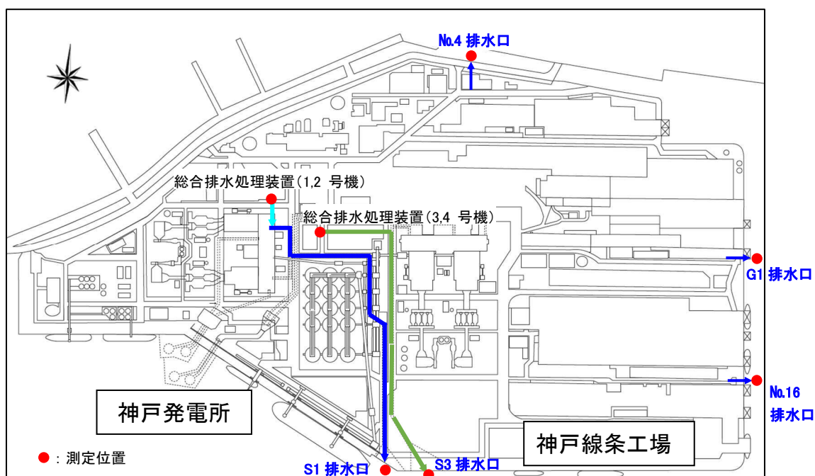
図 8-1 排水口および総合排水処理装置位置図
