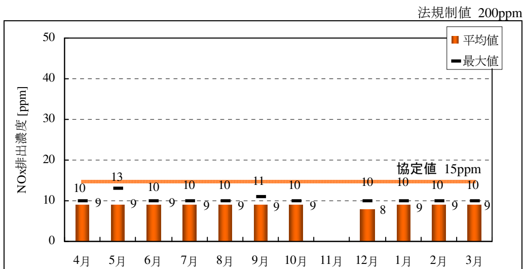
図 6-16 神戸発電所 3 号機の NOx 排出濃度
