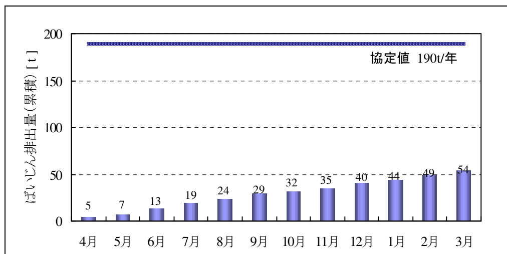
図 6-6 事業場からのばいじん排出量（累積）
