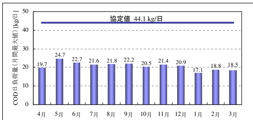
図 8-2 COD の日負荷量 (月間最大値)
