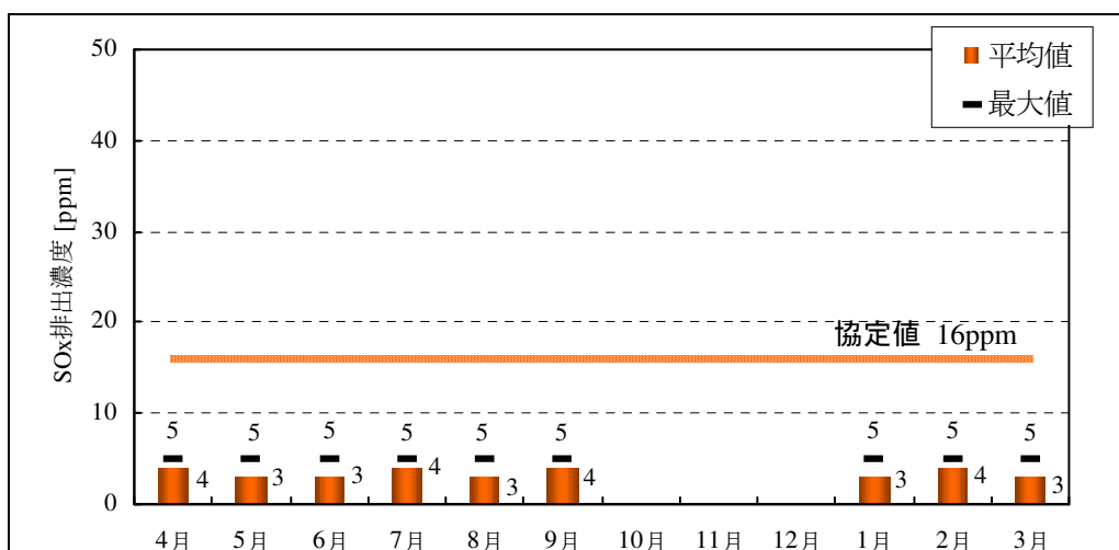
図 6-8 神戸発電所 2 号機の SO x 排出濃度
