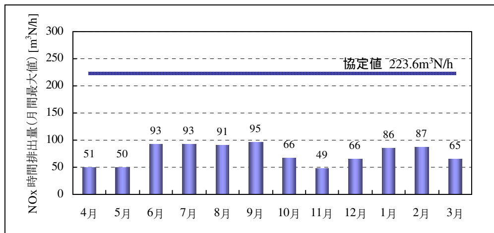
図 6-2 事業場からの NO x 時間排出量 (月間最大値)
