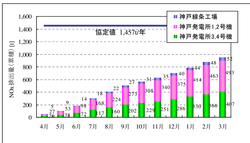
図 3-4 事業場からの NO x 排出量 (累積)
