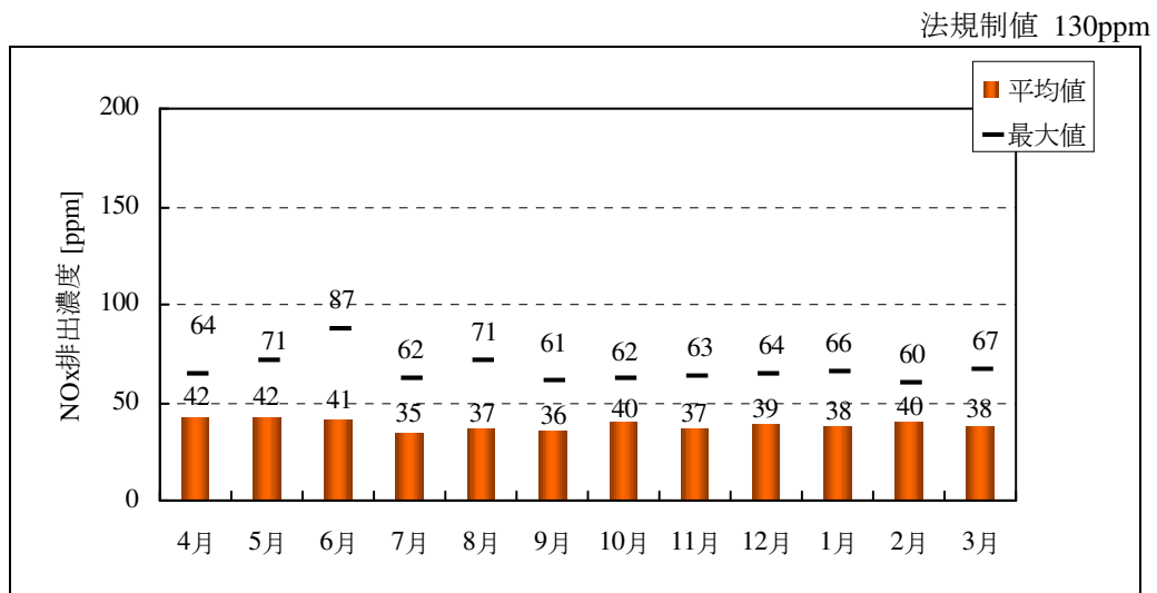
図 6-12 第 7 線材工場加熱炉の NOx 排出濃度
