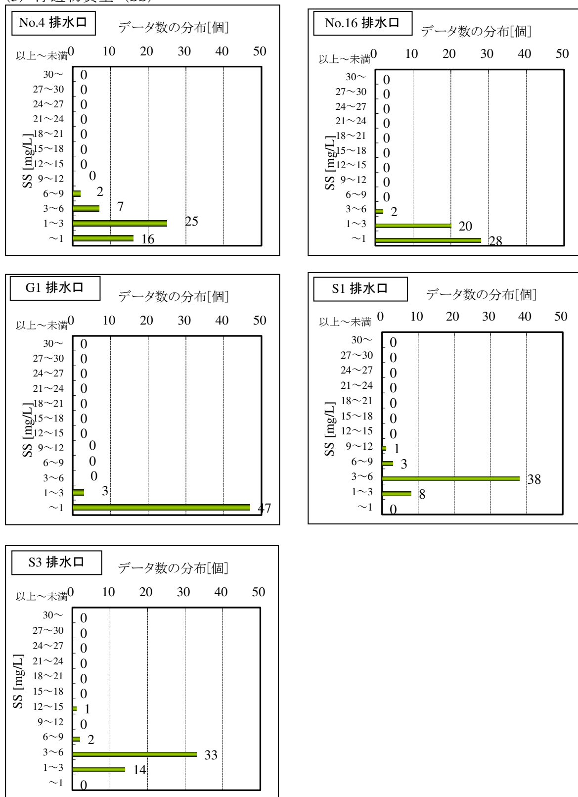
図 4-3 排水水の SS（日平均値）の分布
