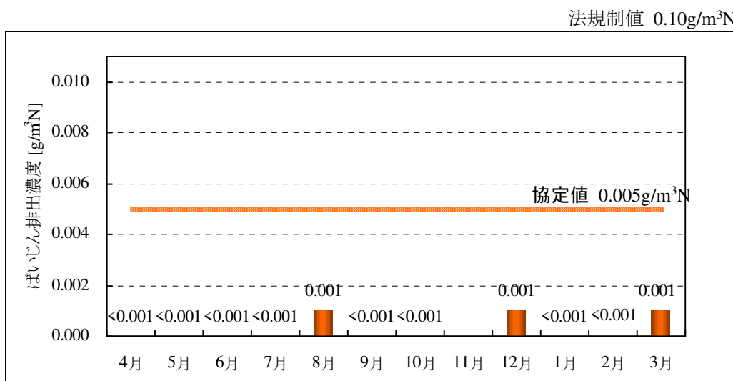
図 6-20 神戸発電所 3 号機のばいじん排出濃度
