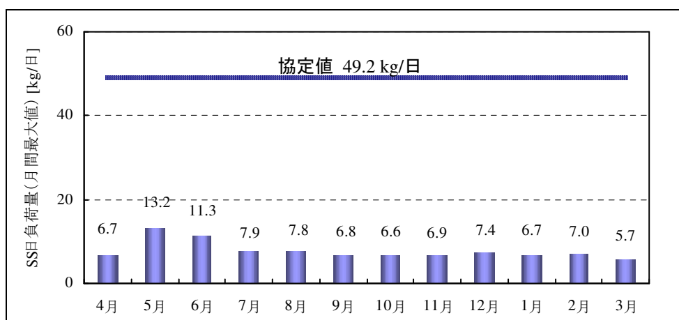
図 8-5 SS の日負荷量 (月間最大値)
