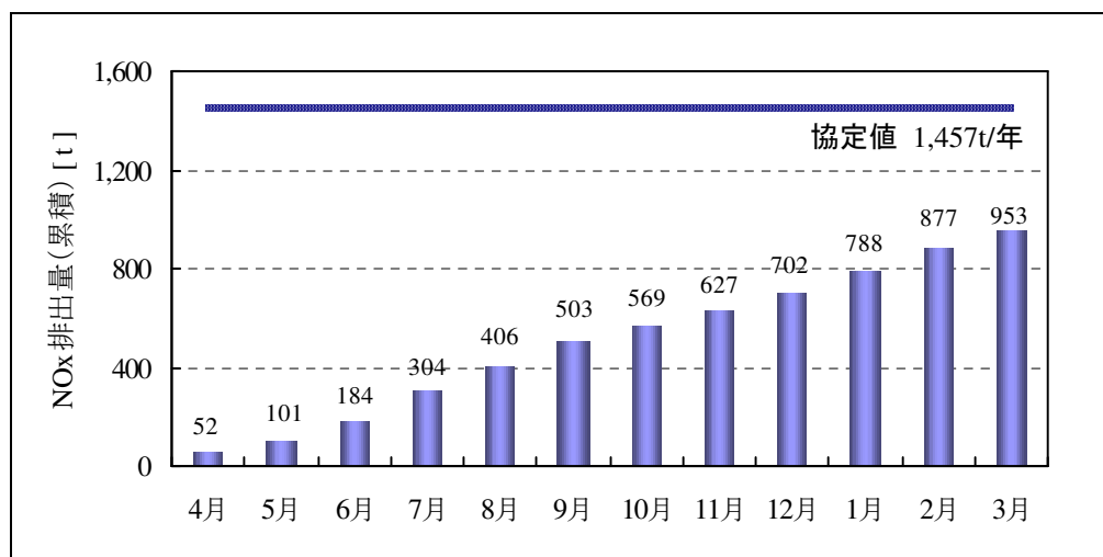
図 6-5 事業場からの NO x 排出量 (累積)
