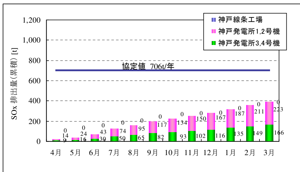
図 3-2 事業場からの SO x 排出量（累積）
