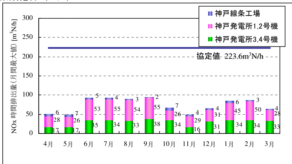
図 3-3 事業場からの NO x 時間排出量 (月間最大値)
