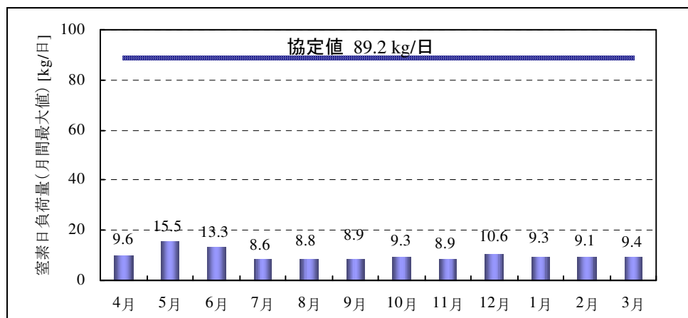
図 8-3 T-N の日負荷量 (月間最大値)
