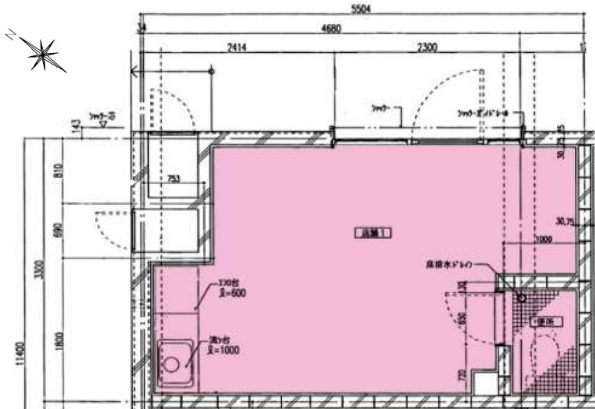
【貸付物件図】 ※単位 mm 寸法は軸心
