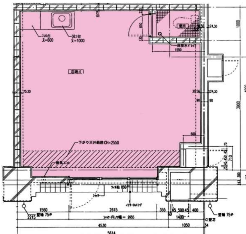
【貸付物件図】 ※単位 mm 寸法は軸心
