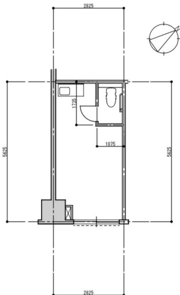
【貸付物件図】 ※単位 mm 寸法は軸心
