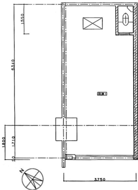
【貸付物件図】 ※単位 mm 寸法は軸心
