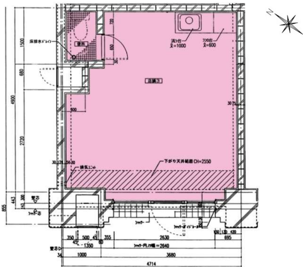
【貸付物件図】 ※単位 mm 寸法は軸心
