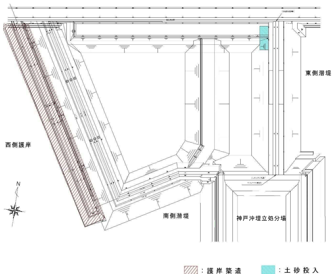
図 I-3-4(1) 護岸築造場所の平面図
