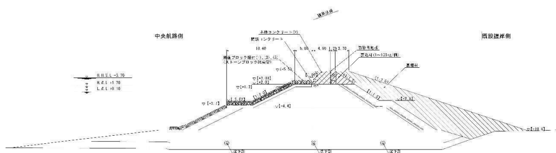
図 I -3-4 (2) 護岸築造場所の断面図
