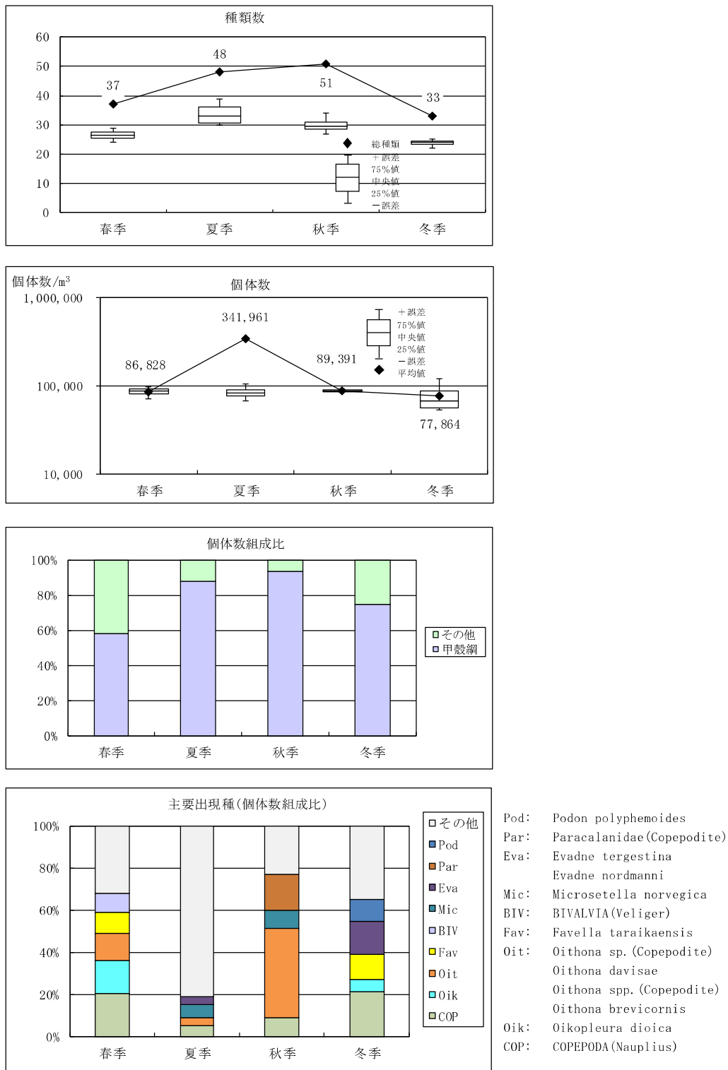
図Ⅱ-6-4 動物プランクトンの調査結果
