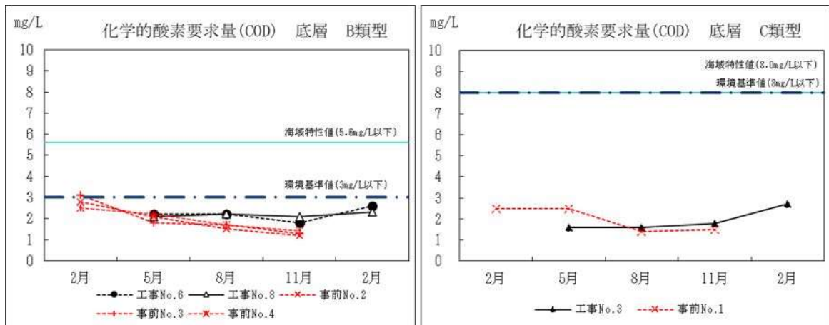
図Ⅱ-3-12 事前調査と工事中の水質の比較 (COD)
