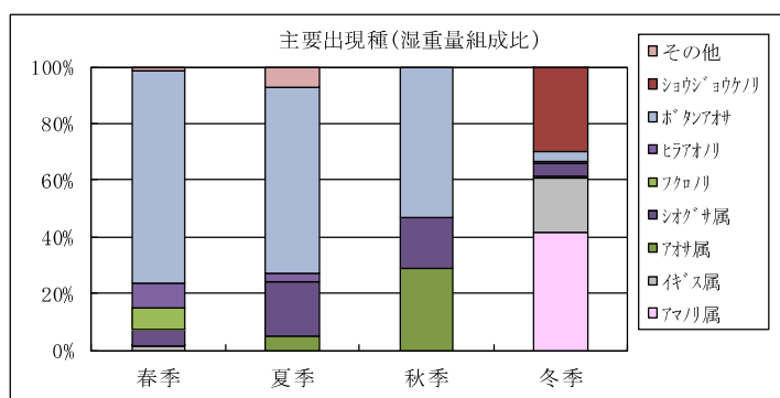
図Ⅱ-6-12 付着生物の調査結果(坪刈り;植物)
