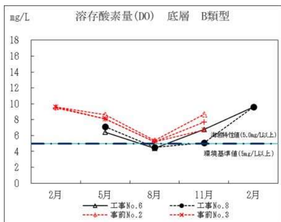
図 II-3-13 事前調査と工事中の水質の比較 (DO)
