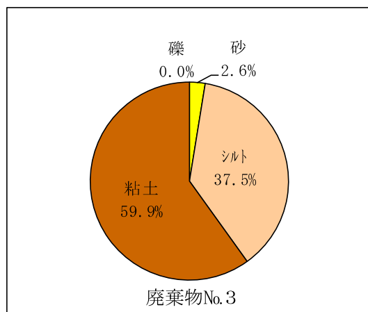
図 II-4-2 底質(粒度組成)の水平分布
