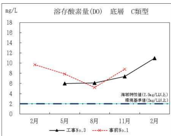
図 II-3-13 事前調査と工事中の水質の比較 (DO)
