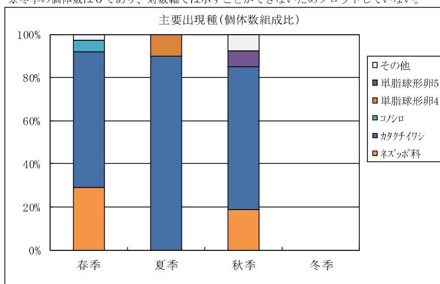
図Ⅱ-6-5 魚卵の調査結果
