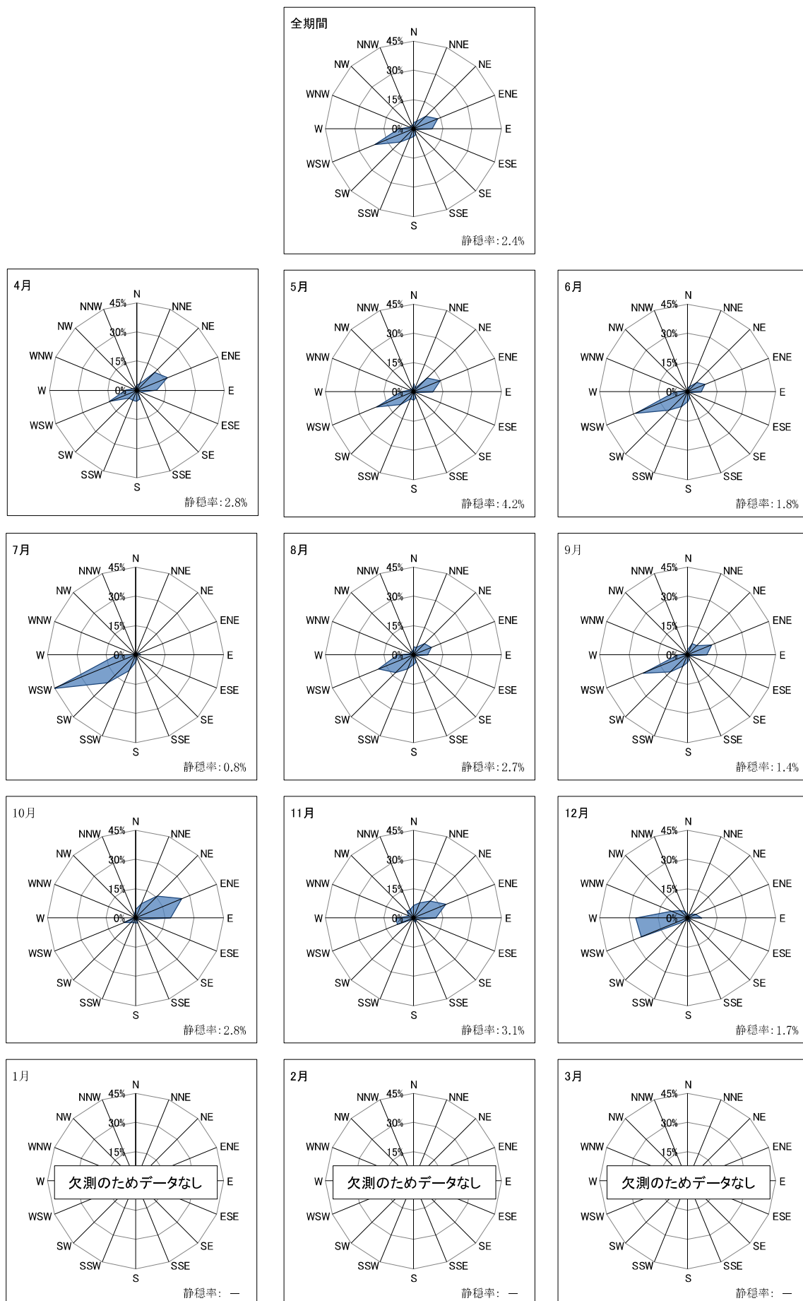
図Ⅱ-1-2 風配図
