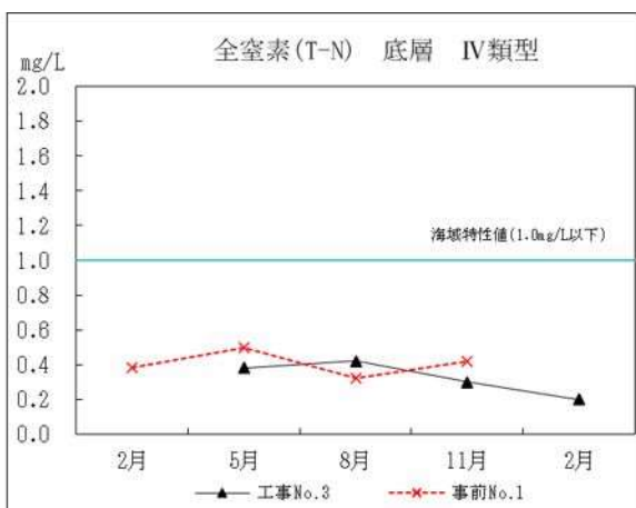
図Ⅱ-3-14 事前調査と工事中の水質の比較 (T-N)
