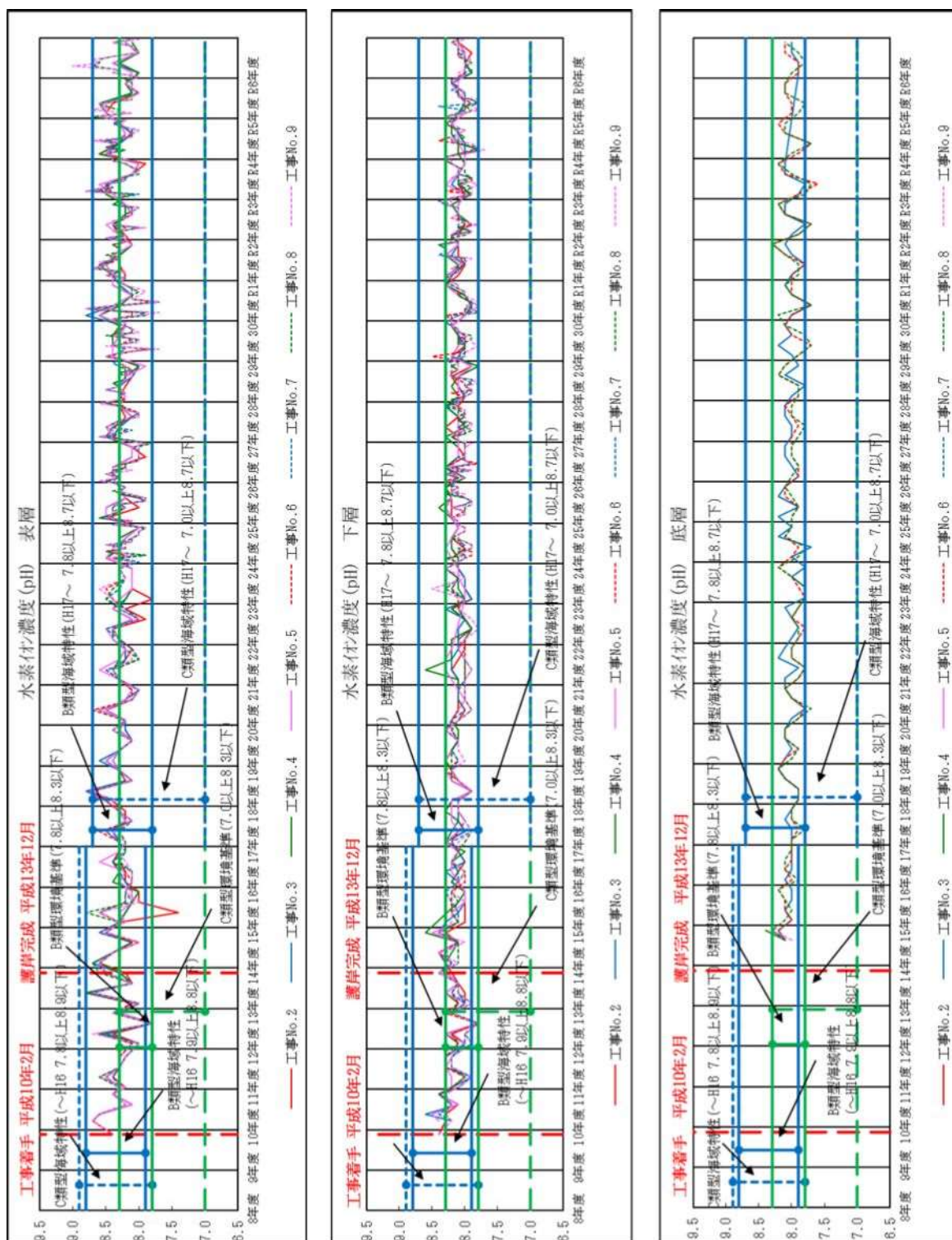
図Ⅱ-3-17 工事中の水質の経年変化 (pH)
