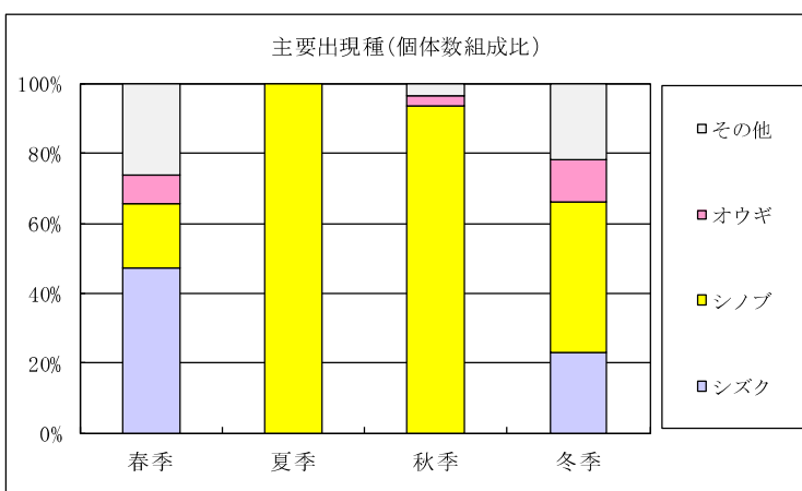
図 II-6-7 底生生物の調査結果
