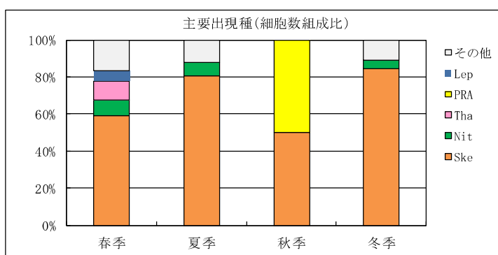
図Ⅱ-6-3 植物プランクトンの調査結果
