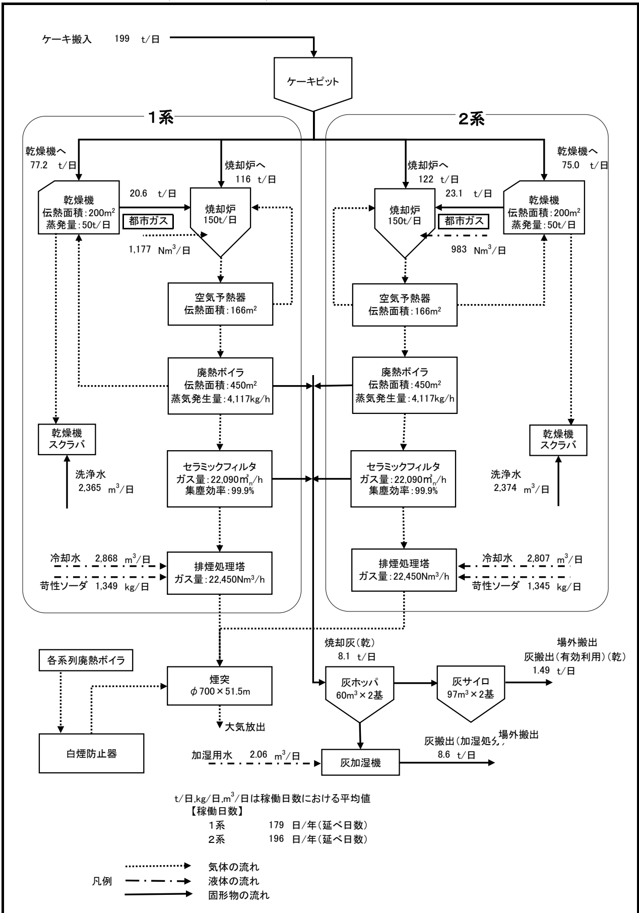
焼却施設フローチャート(稼働日数平均)
