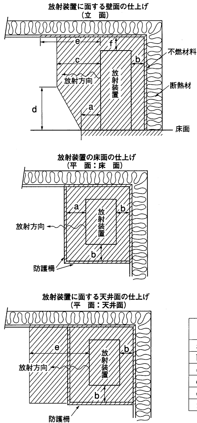
図1 遠赤外線放射装置の離隔距離等及び周辺の仕上げ
