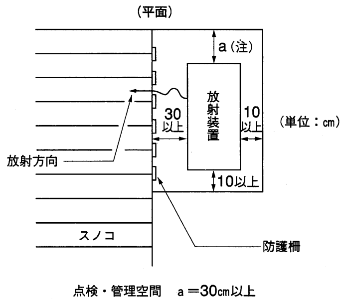
図3 点検・管理空間（平面図）
