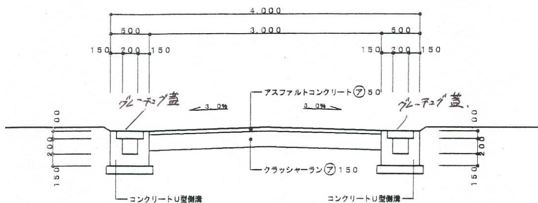
標準横断面図 1/50
