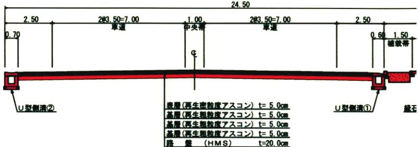
⑤－⑤断面図
