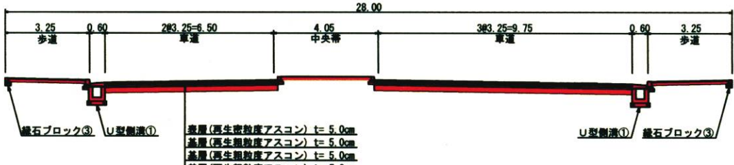
③－③断面図
