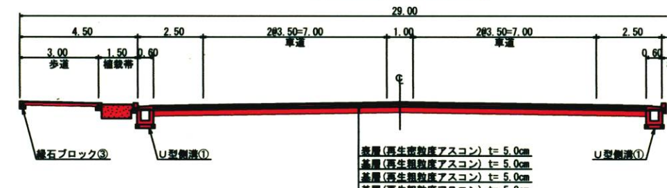
⑥－⑥断面図
