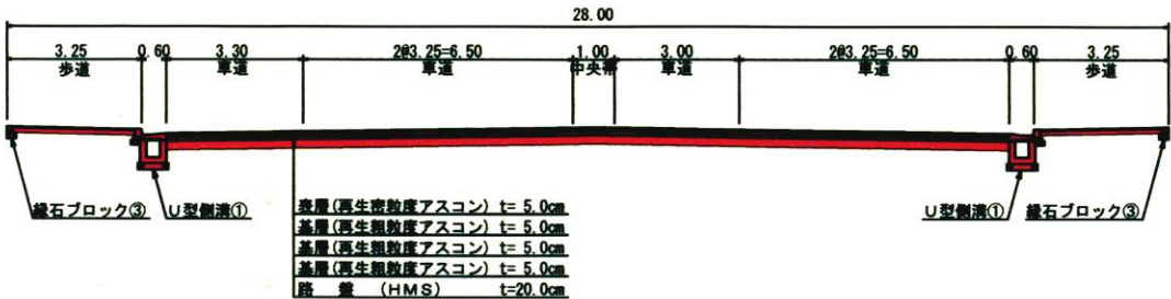
②－②断面図
