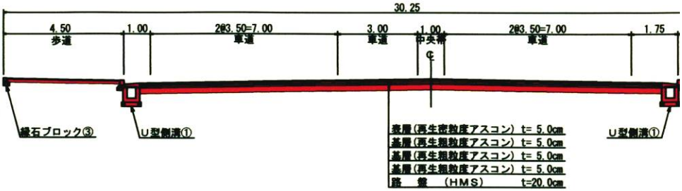
④－④断面図
