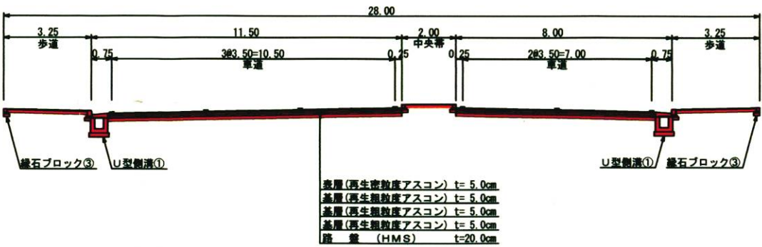
②－②断面図
