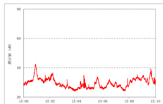
St2 地点
