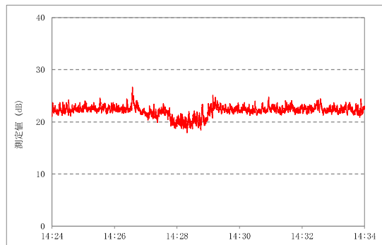
中間変電所
