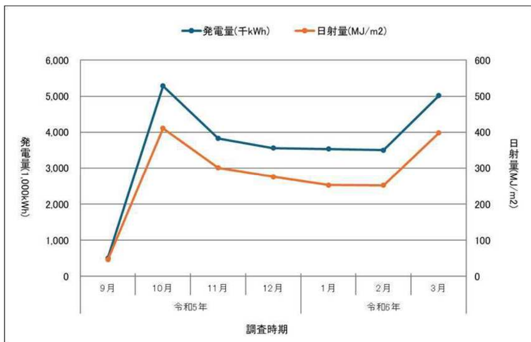
図 3.7-1 施設稼働後の発電量及び日射量
