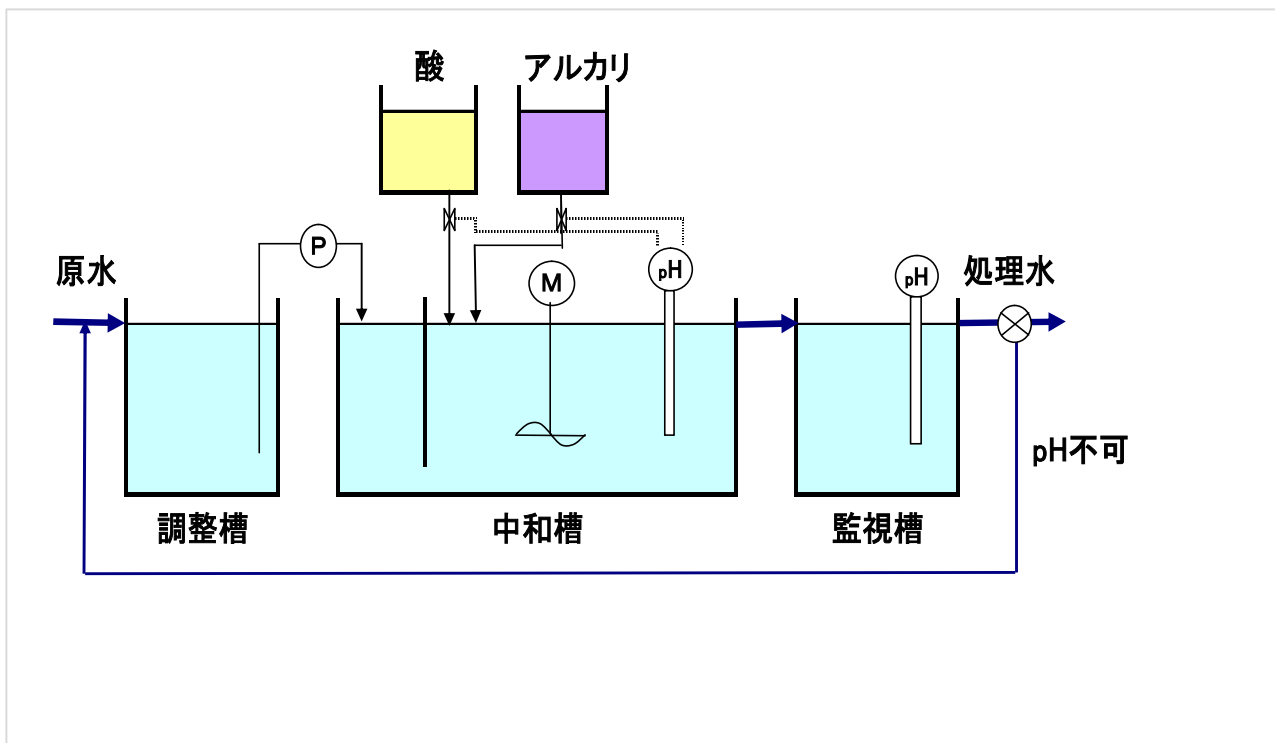
図 4 中和処理フロー
