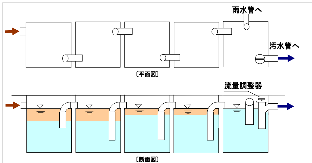
図1 油水分離槽(ガソリンスタンド向け)
