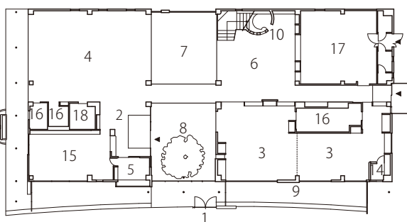
1階平面図
