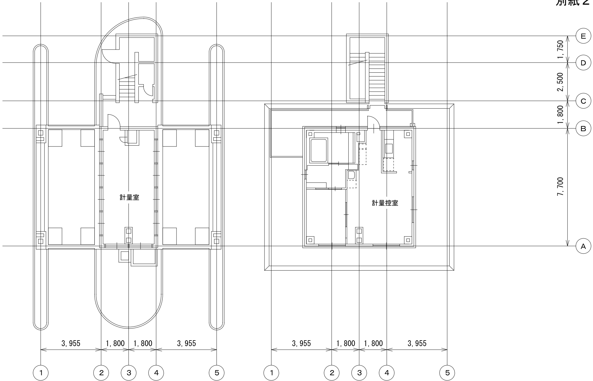
計量棟 1階
