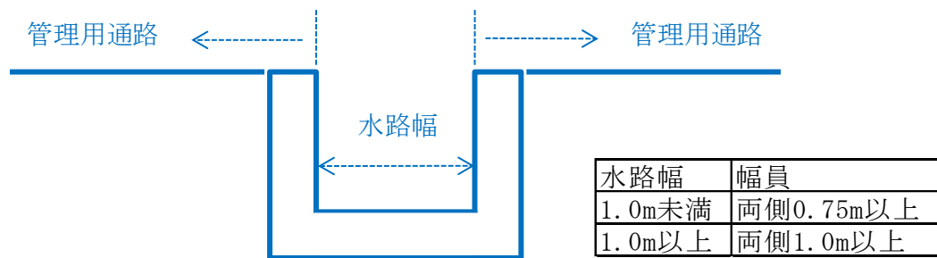
水路幅と管理用通路の幅員に関する標準構造図
