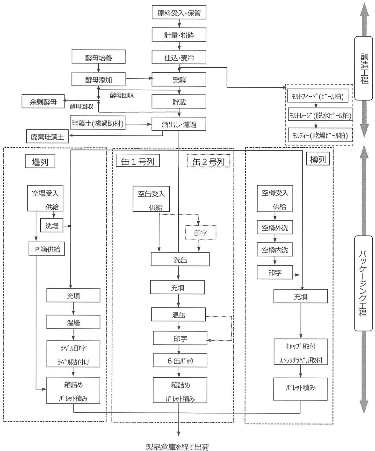
図1 ビール製造工程
