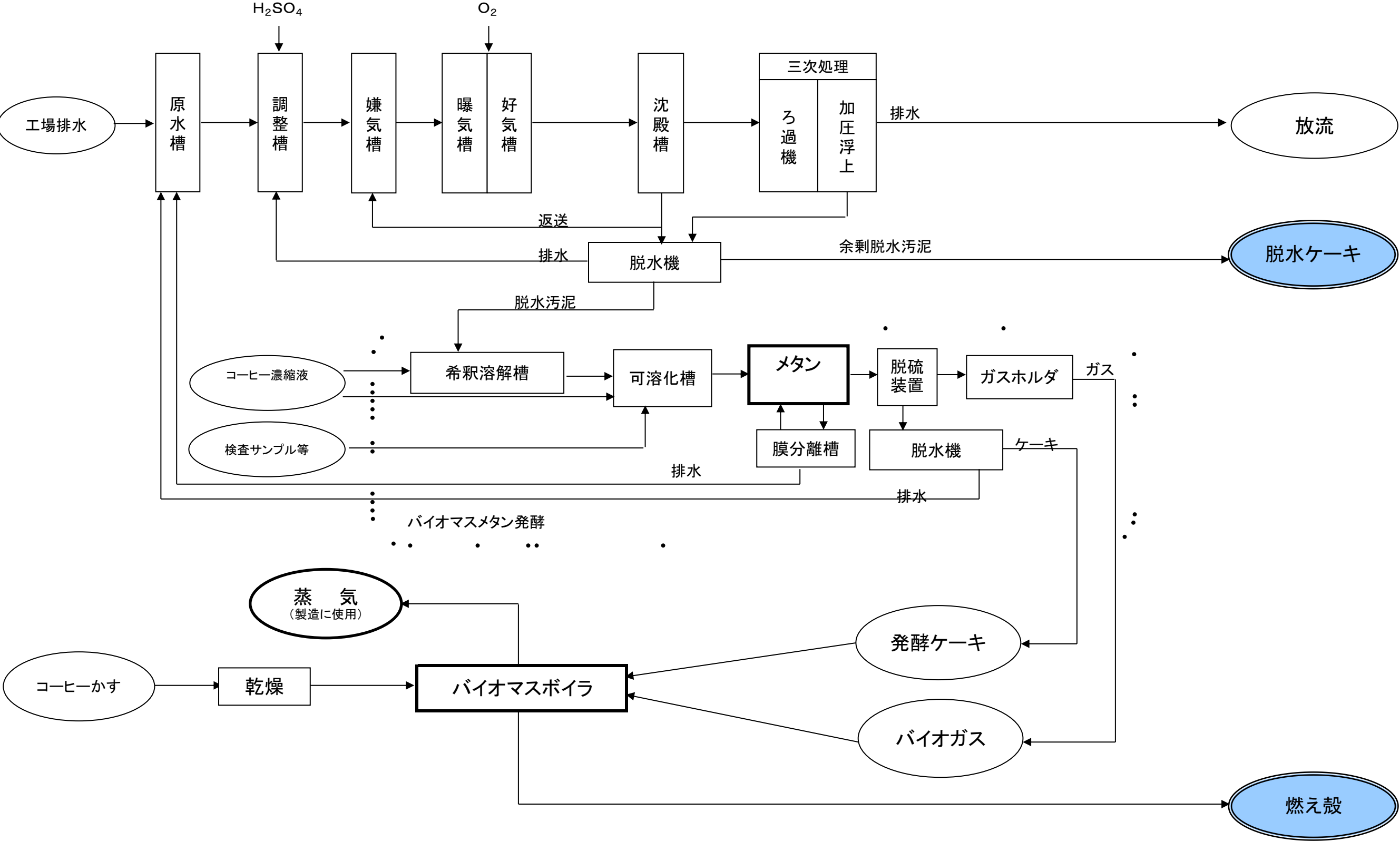
図2 排水フロー
