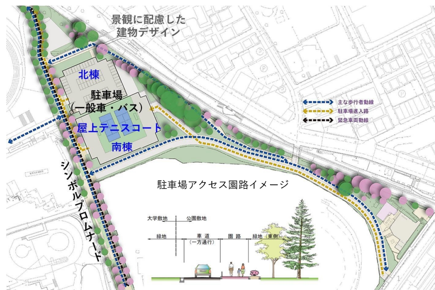
【駐車場・アクセス園路 計画図】
