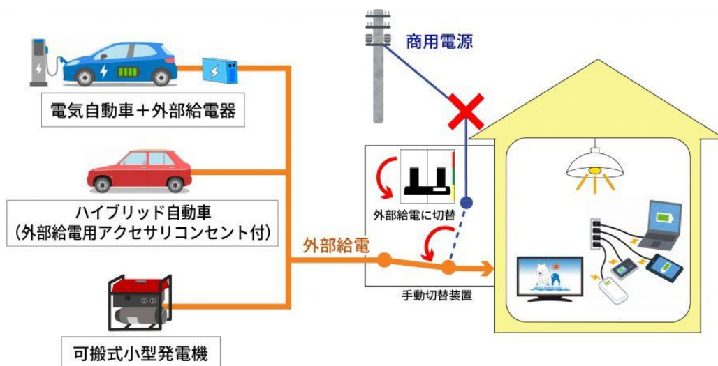
図 25 外部給電神戸モデルのイメージ図
