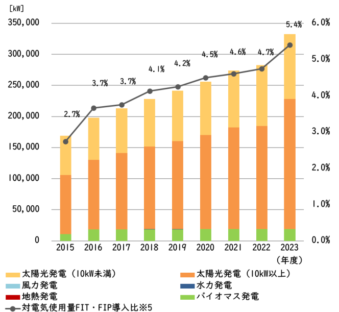
図 11 再生可能エネルギー導入実績
