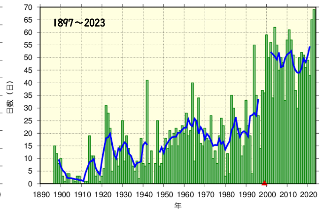
図 33 神戸の年間熱帯夜日数
