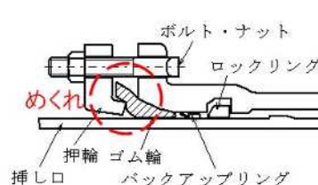
図 接合不良の例
