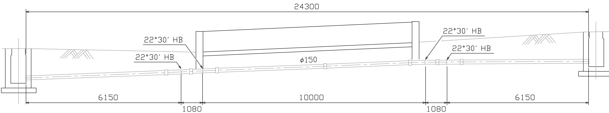
\phi 150 電送管縦断面図
