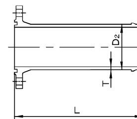
G X 形 短管 2 号
