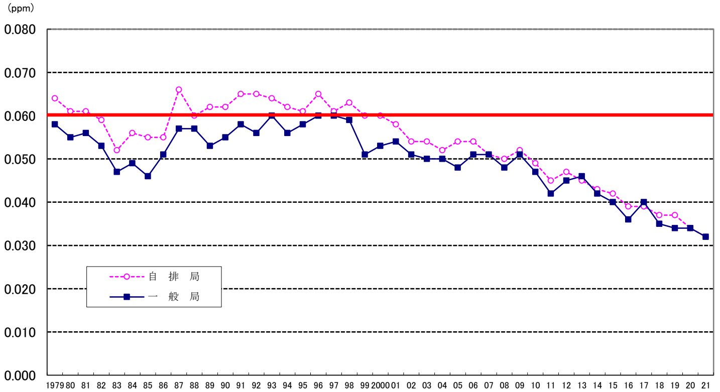
図2 二酸化窒素の年間98%値(上位3局平均値)の経年変化
