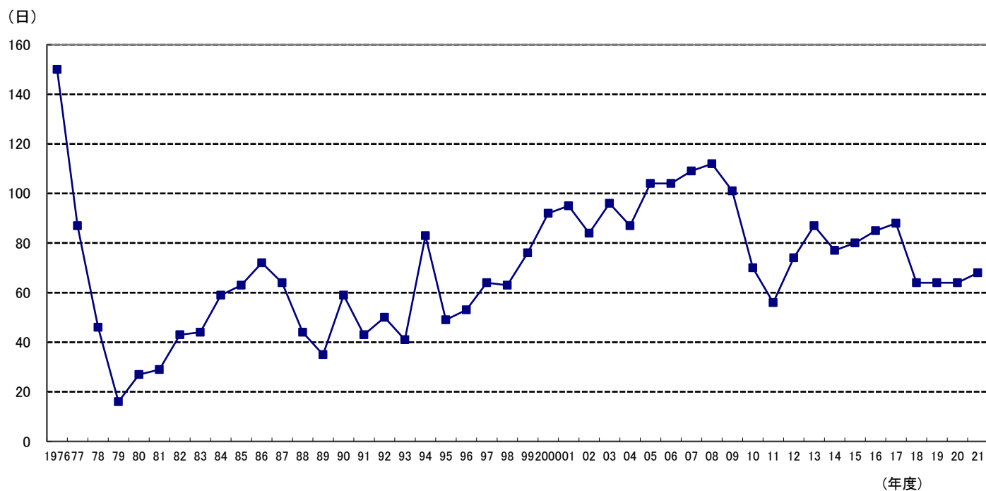
図7 昼間の1時間値が0.06ppmを超えた日数の経年変化(光化学オキシダント)
