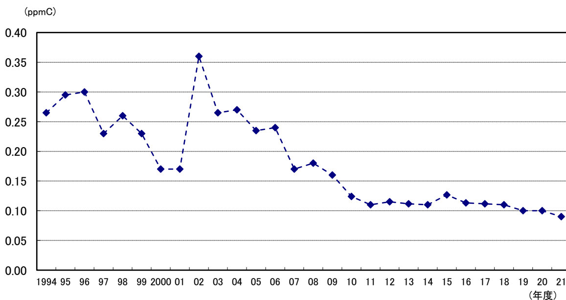
図9 非メタン炭化水素の経年変化(午前6時から9時までの3時間の年平均値)
