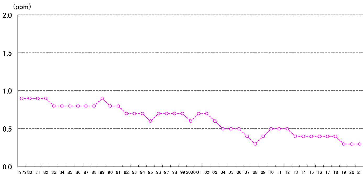
図 3 一酸化炭素の年平均値の経年変化
