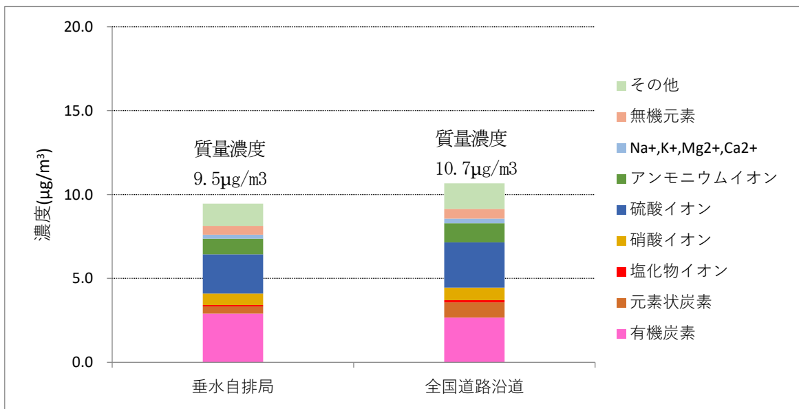
図6-2 PM2.5成分分析結果 (垂水自排局)
