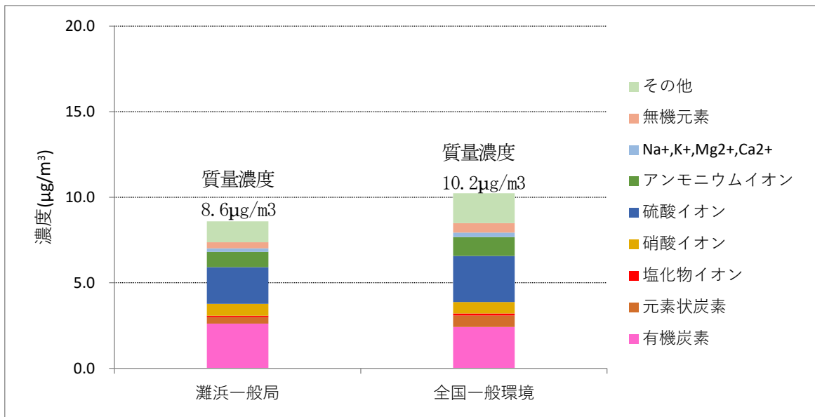
図6-1 PM2.5成分分析結果 (灘浜一般局)
