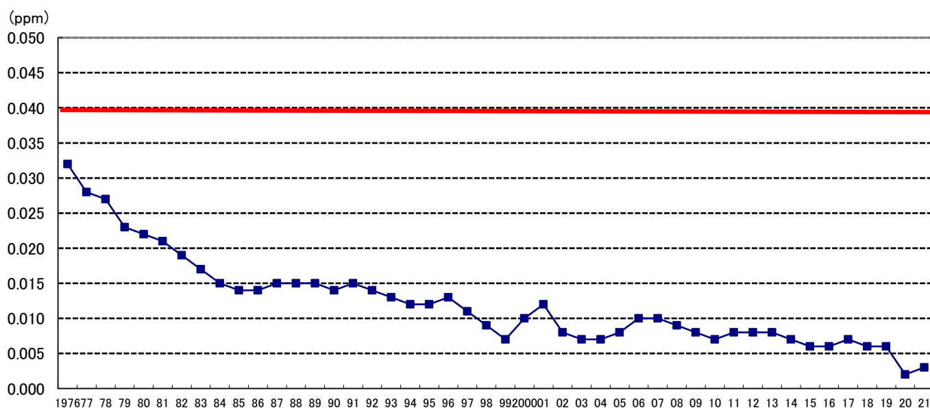
図1 二酸化硫黄の2%除外値（平均値）の経年変化
