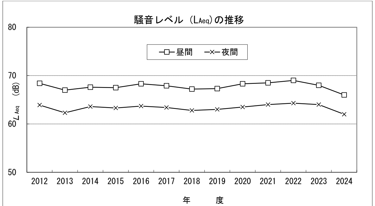
図 2.2 道路交通騒音の経年変化
