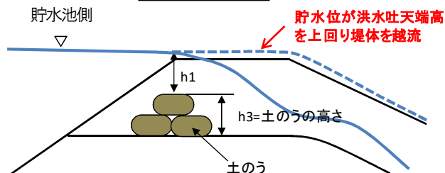
洪水吐流入部に土のうを積んだ場合
