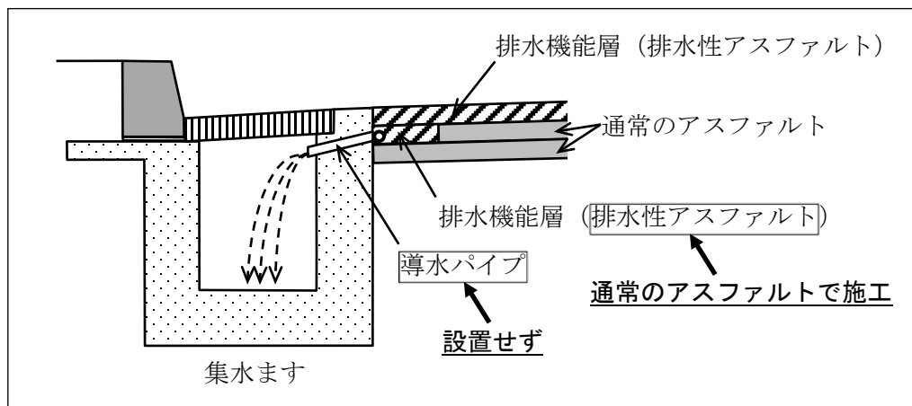
排水性アスファルト舗装のイメージ
