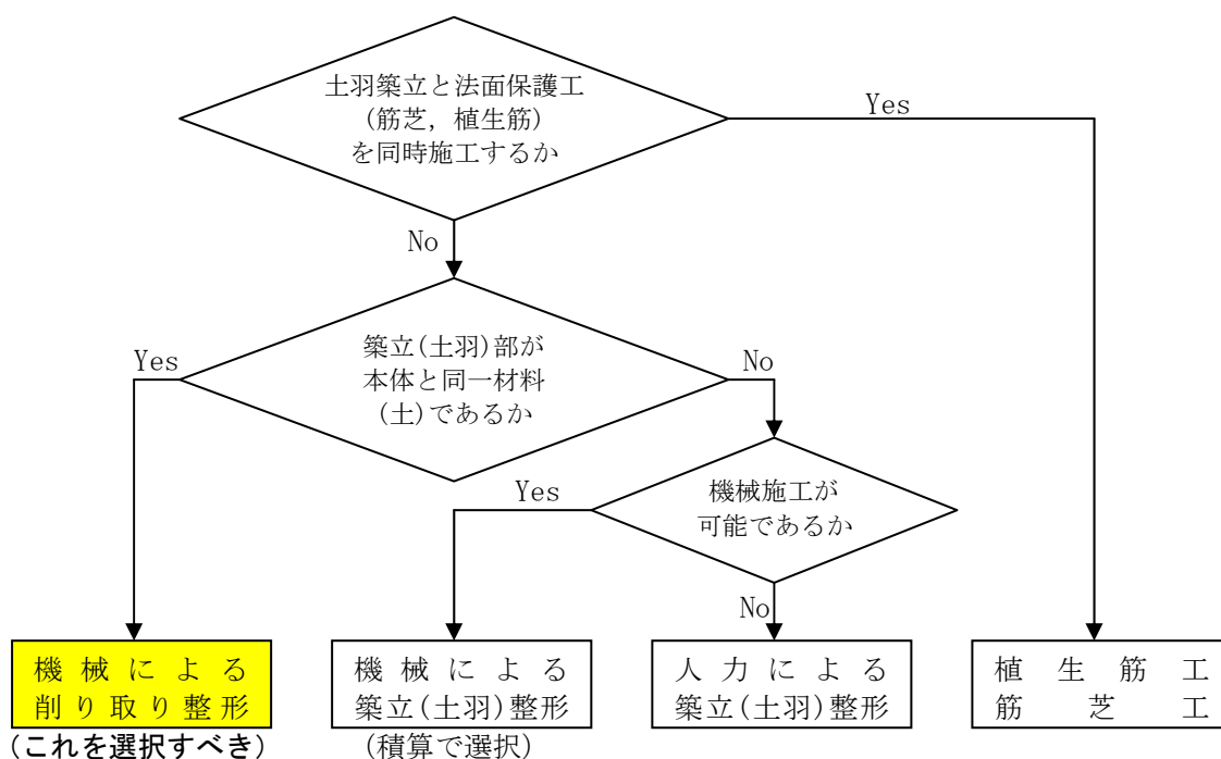
盛土法面整形工の工法選定フロー
