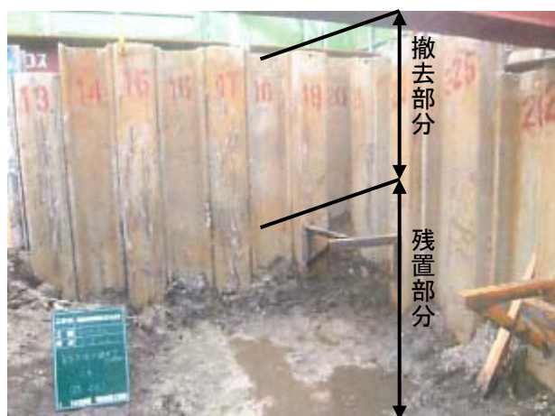
鋼矢板設置状況
