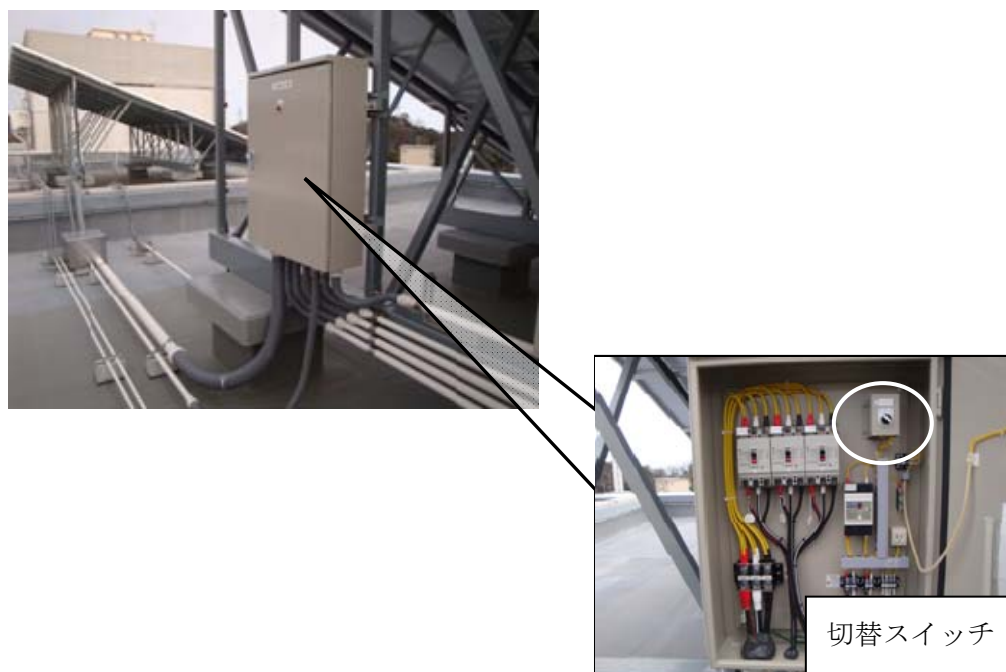
交流集合盤と自立運転切替スイッチ（例）
