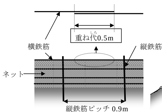
しがら工 正面図
