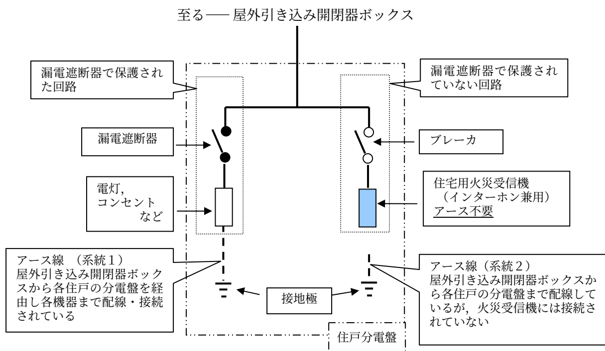
各住戸の分電盤の接続概要図
