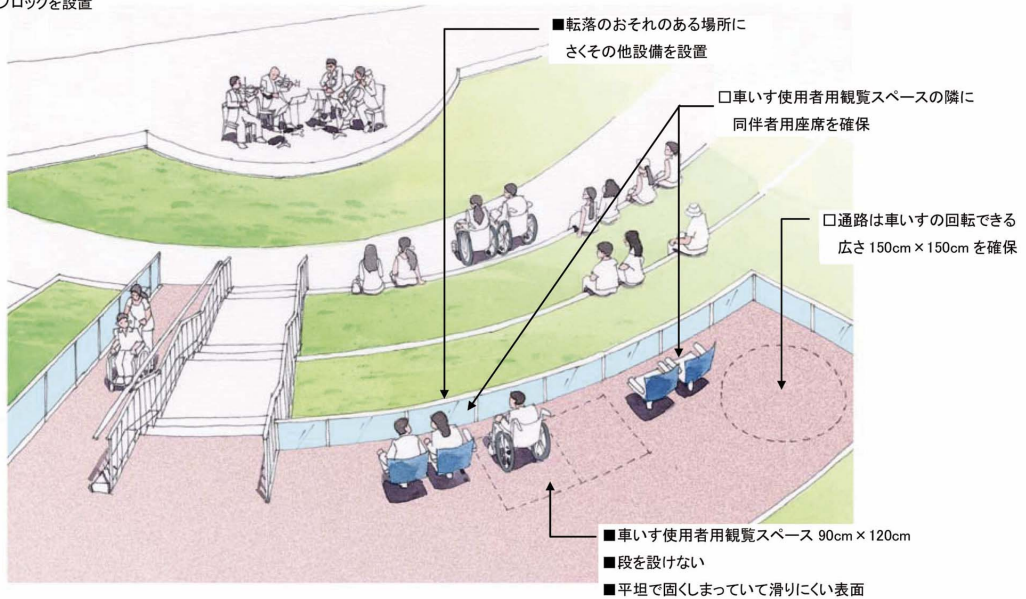
図 4-1 野外劇場の整備例
