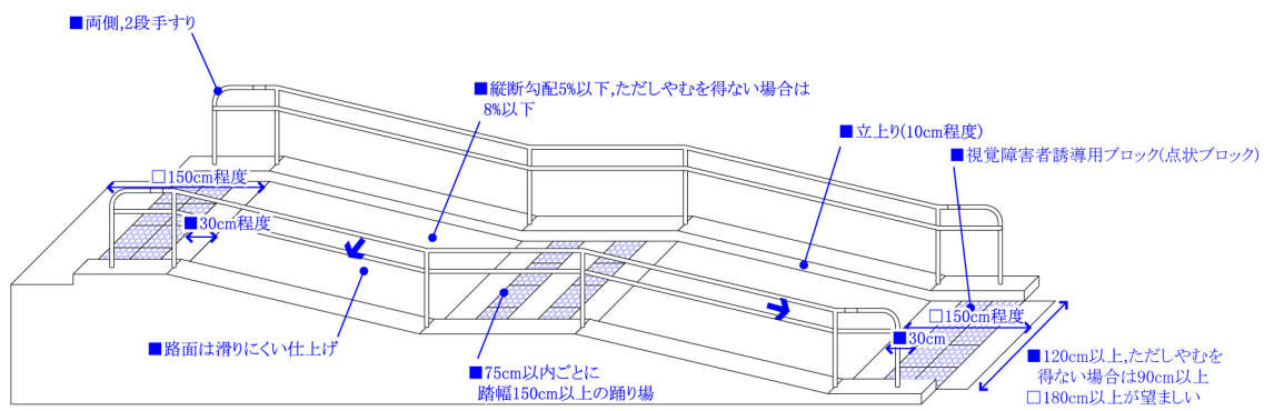
図 1-7 傾斜路の整備例
