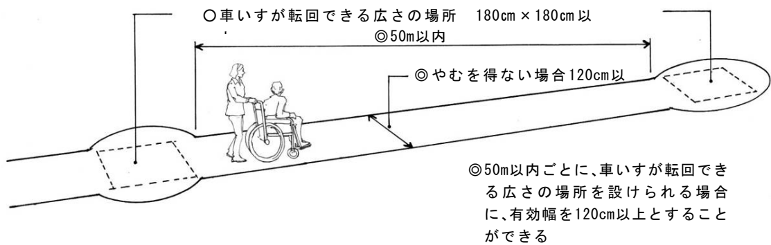
図 1-5 通路の整備例
