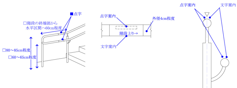
図 1-6 階段の整備例
