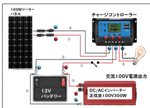
手作りソーラー発電システム
