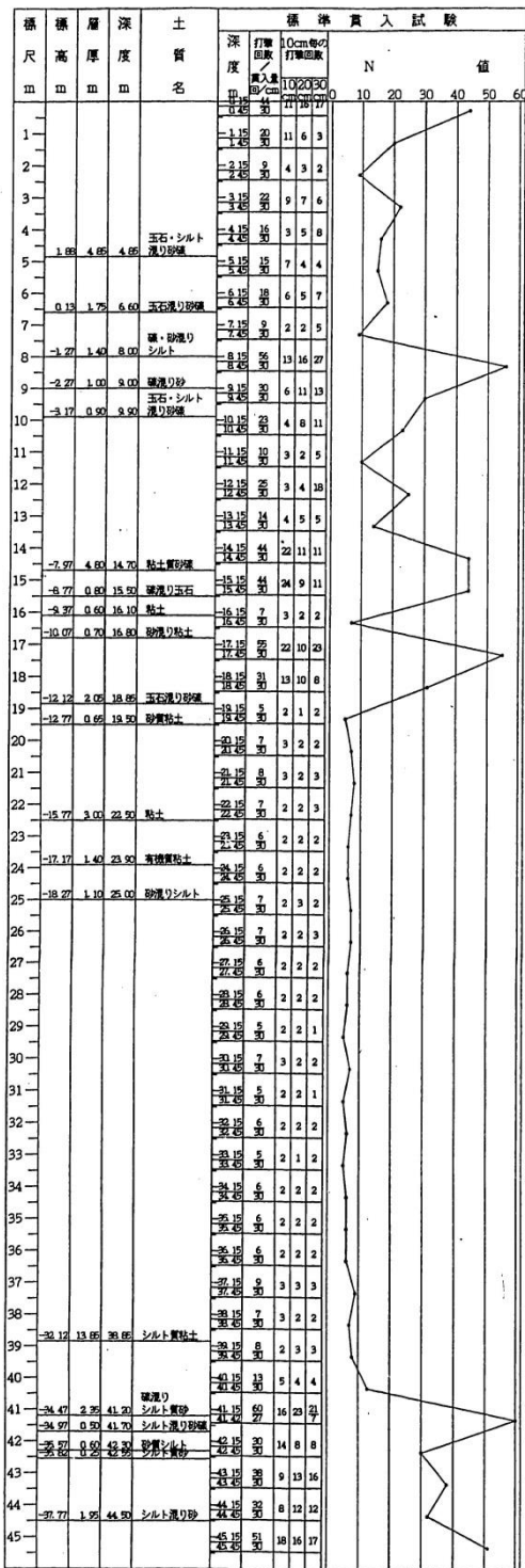
図-2 土質柱状図
