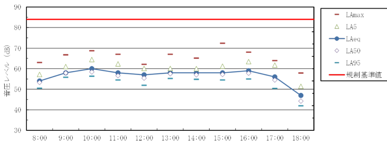
図Ⅱ-2-3 騒音レベルの時間変化（令和7年2月6日）
