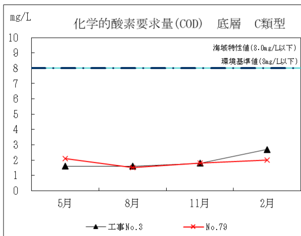
図Ⅱ-3-8 工事中の水質の年間推移 (COD)
