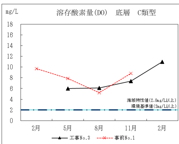
図Ⅱ-3-13 事前調査と工事中の水質の比較 (DO)
