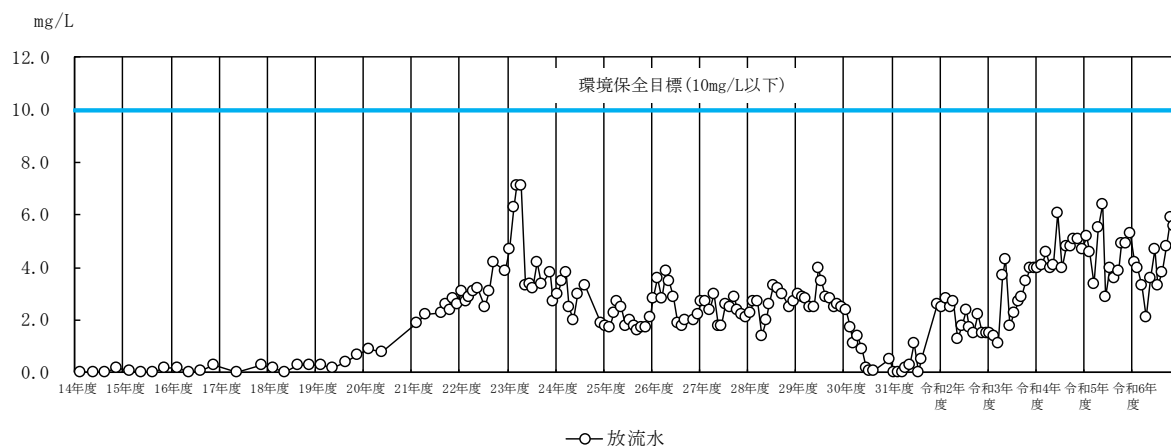
図Ⅱ-3-35 放流水中の溶解性マンガン濃度の経年変化
