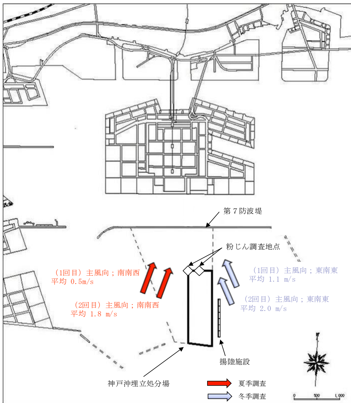
図Ⅱ-1-3 粉じん量調査地点位置図
