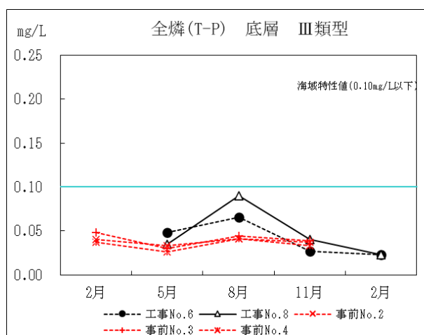
図Ⅱ-3-15 事前調査と工事中の水質の比較 (T-P)
