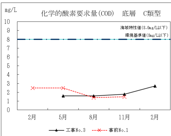
図 II-3-12 事前調査と工事中の水質の比較 (COD)
