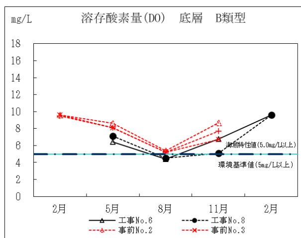
図Ⅱ-3-13 事前調査と工事中の水質の比較 (DO)
