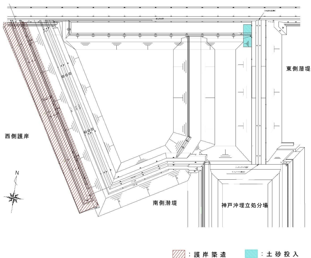
図 I -3-4(1) 護岸築造場所の平面図
