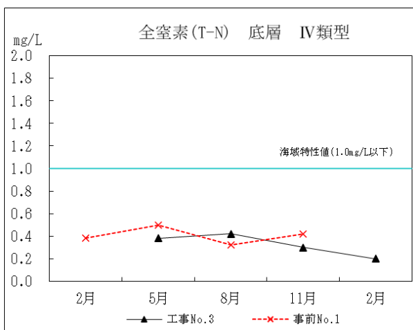
図Ⅱ-3-14 事前調査と工事中の水質の比較 (T-N)
