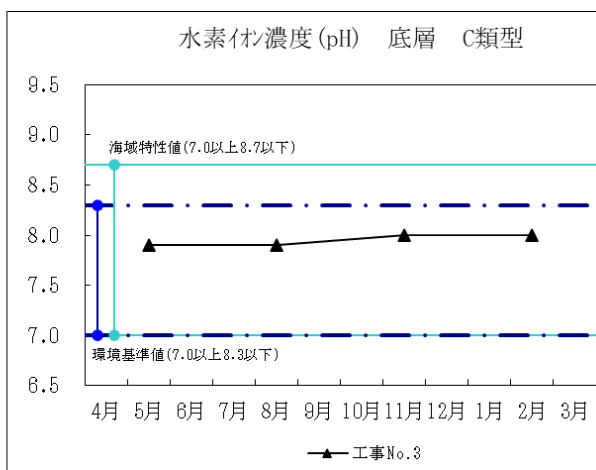
図Ⅱ-3-7 工事中の水質の年間推移 (pH)
