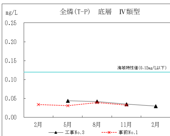
図Ⅱ-3-15 事前調査と工事中の水質の比較 (T-P)
