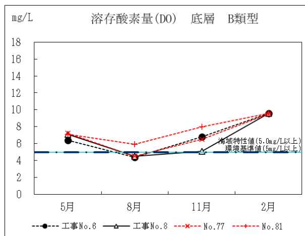
図Ⅱ-3-9 工事中の水質の年間推移(DO)
