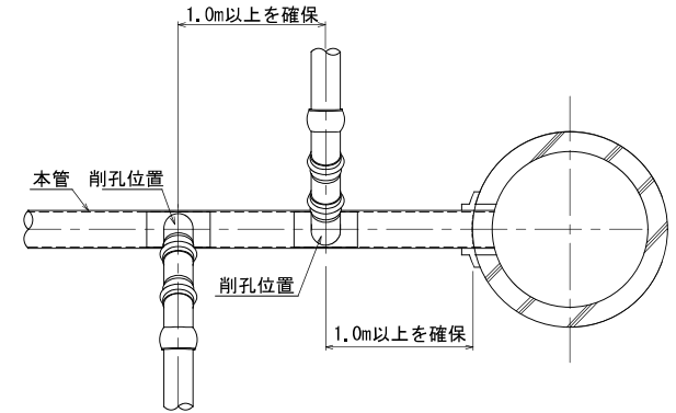
取付管の削孔位置
