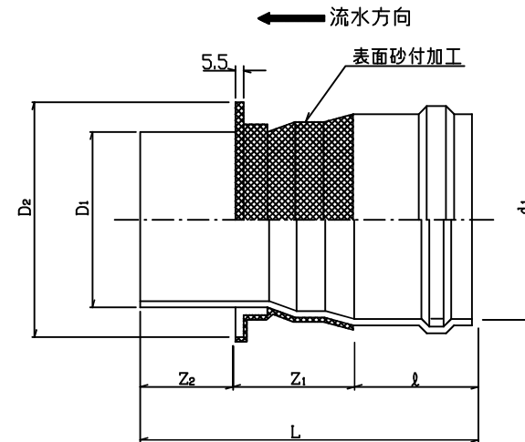
受差兼用枝付支管
