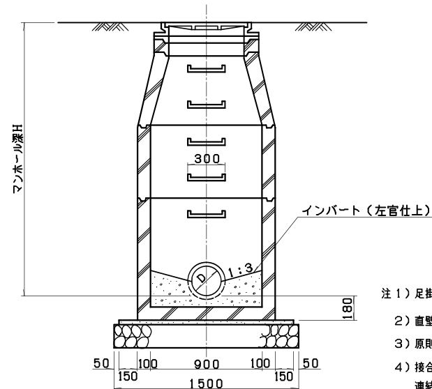
B-B 断面図
