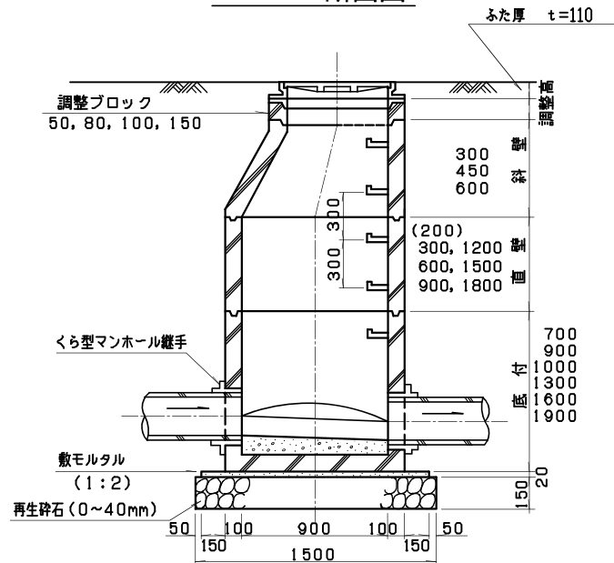
A-A 断面図
