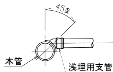
浅埋用支管
