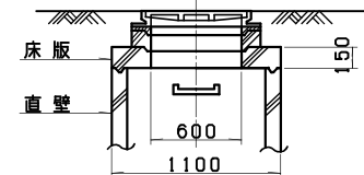
B-B 断面図
