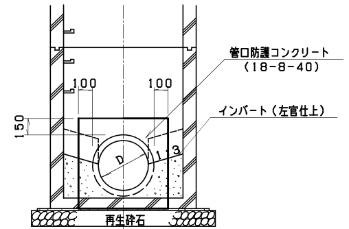
横断面図
