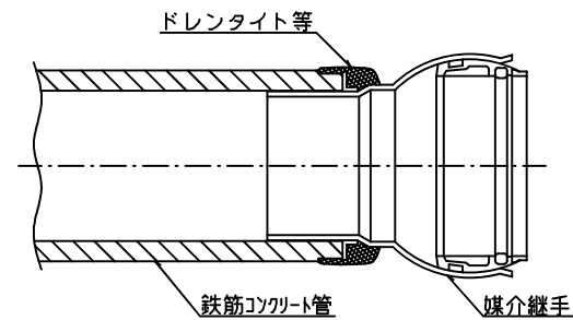
差口側の場合
