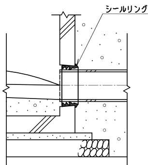
シールリング詳細図
