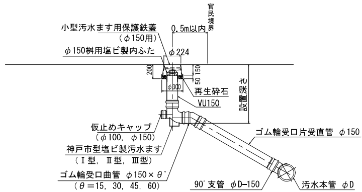
本管が円形管の場合 (下水道設計標準図 P45, P47)
