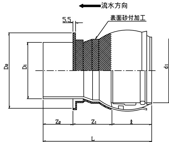
受差兼用枝付自在支管
