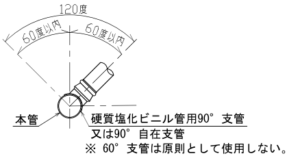
取付管用支管の取付位置 (下水道設計標準図 P45)
