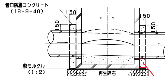
縦断面図
