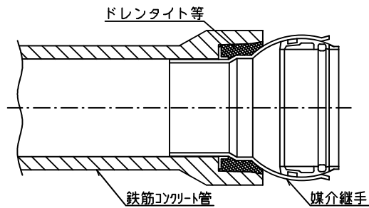
受口側の場合
