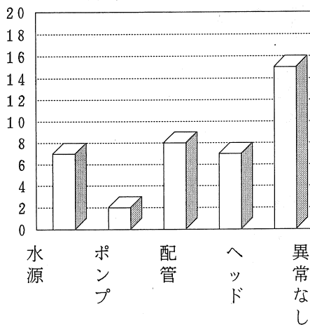
スプリンクラー設備 (設置29対象)
