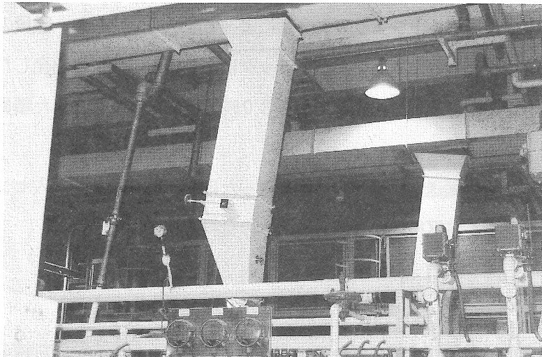
菓子パン製造ラインの排気ダクトの破損
