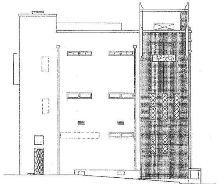
西立面図
