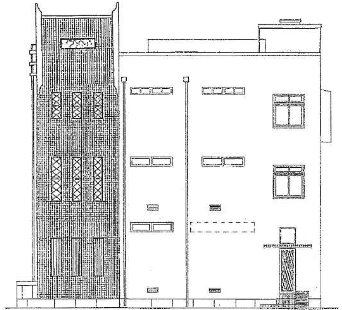
東立面図
