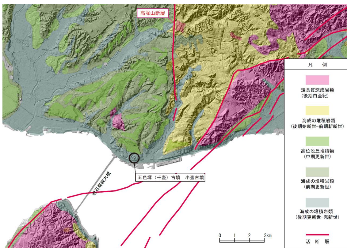
図 2-5 地質図
