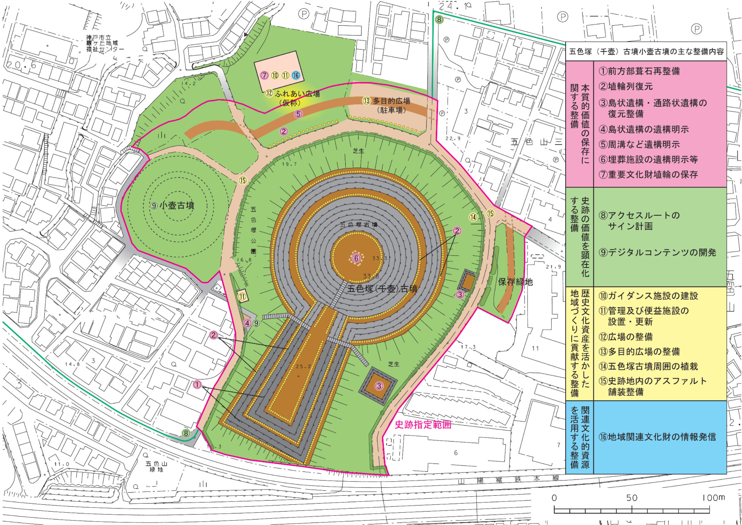
図 10-2 全体計画図
